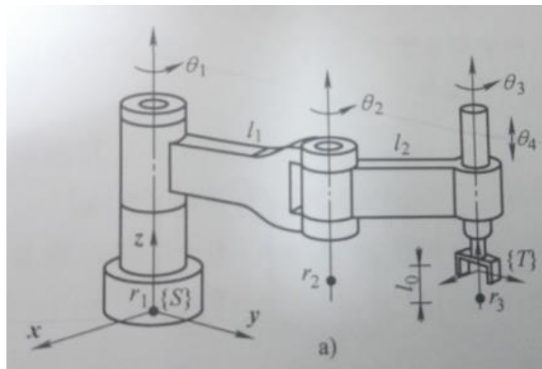
SCARA机器人结构简图
