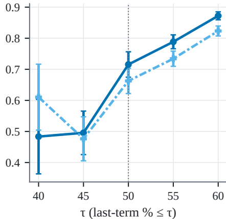
(b) PR-AUC
