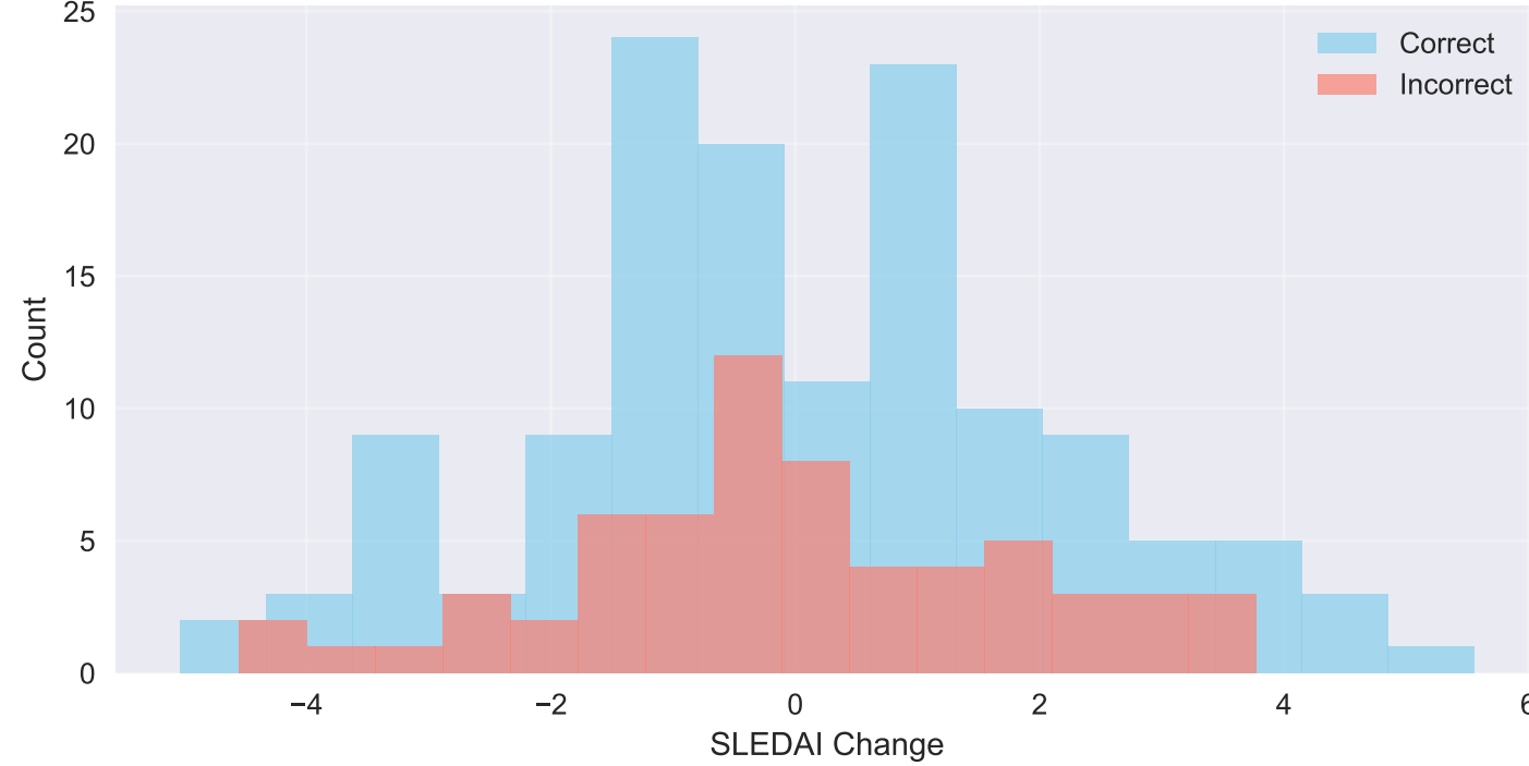
TAGT: Accuracy vs SLEDAI Change
