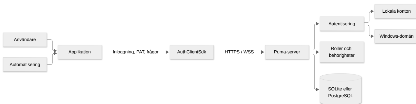
Figur 1: Översikt över Pumas systemarkitektur.
