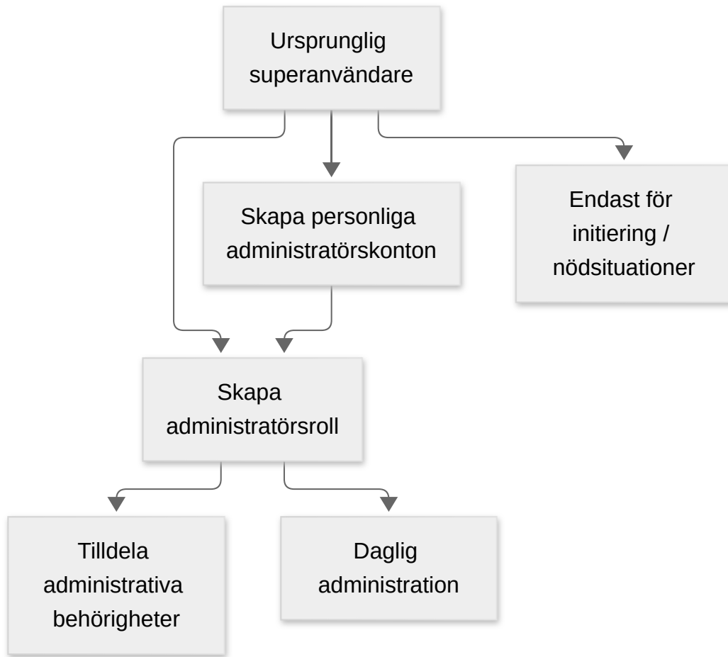
Figur 5: Rekommenderad modell för initiering och daglig administration.
