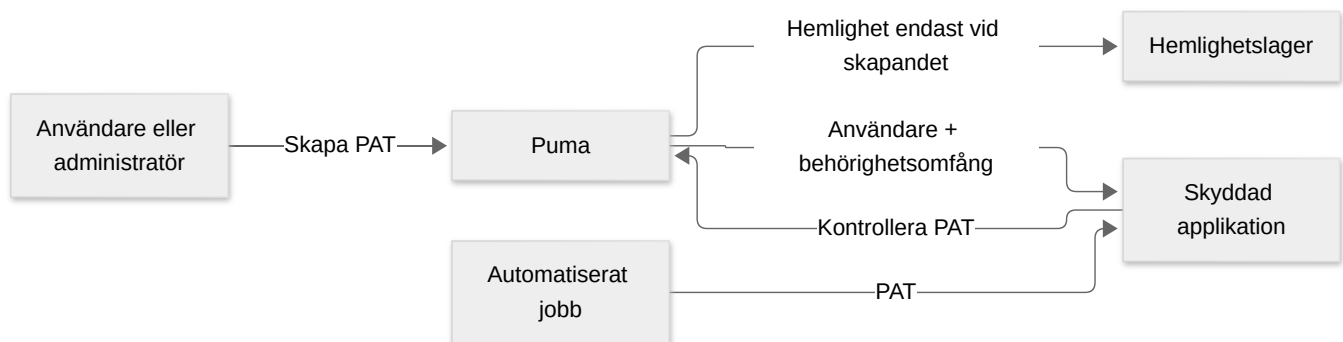
Figur 15: Skapande, lagring och användning av en PAT.
