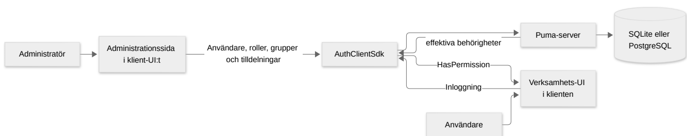
Figur 3: Central administration och användning av behörigheterna i applikationen.
