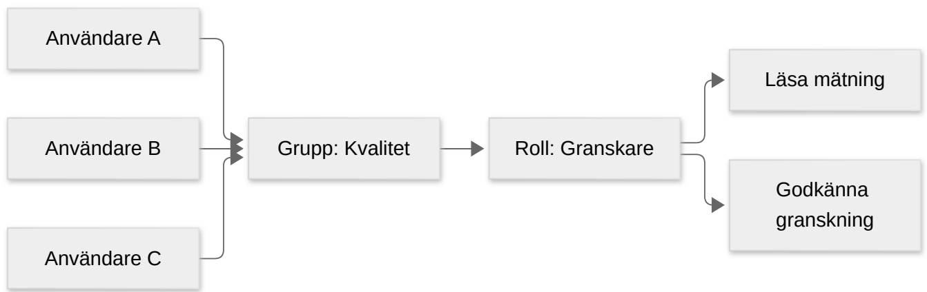
Figur 10: Gemensam behörighetstilldelning via en grupp.
