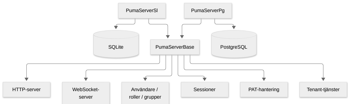
Figur 2: Gemensam serverbas och databasspecifika varianter.
