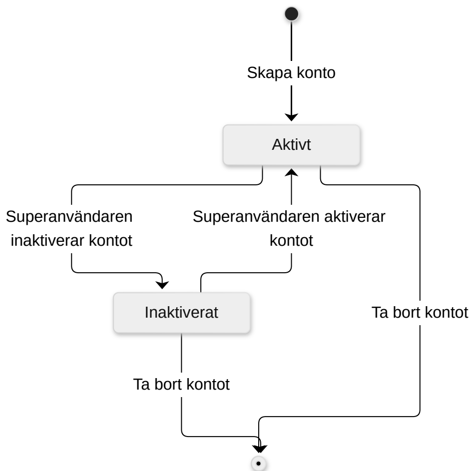
Figur 19: Kontostatus och övergångarna som superanvändaren utlöser.
