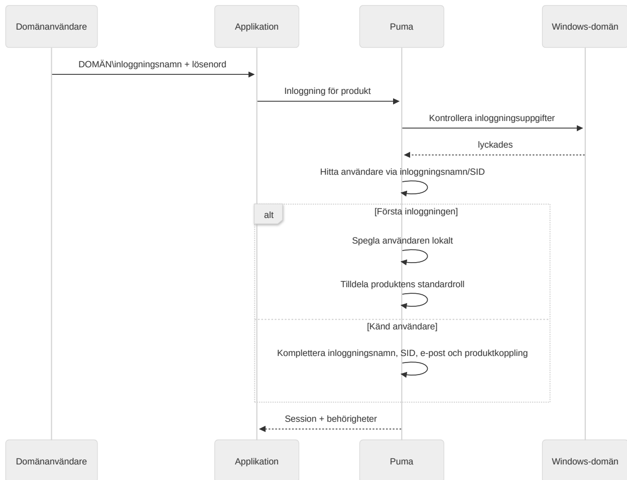
Figur 14: Inloggning av en Windows-domänanvändare via Puma.
