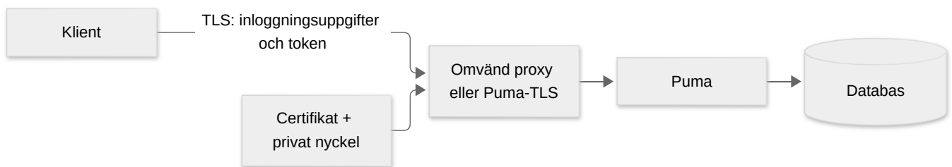
Figur 8: TLS-skyddad transport mellan klienten och Puma.
