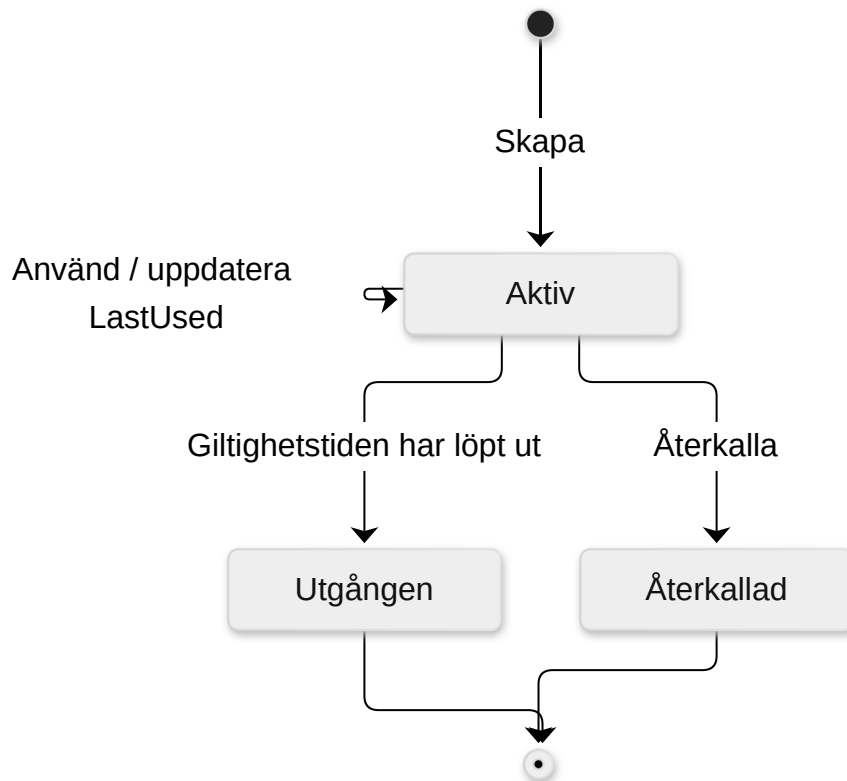
Figur 16: Tillstånd i en PAT:s livscykel.
