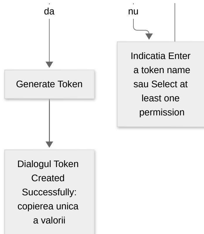
Figura 4: Crearea unui jeton personal de acces pe pagina de profil – valoarea jetonului este afișată o singură dată.
