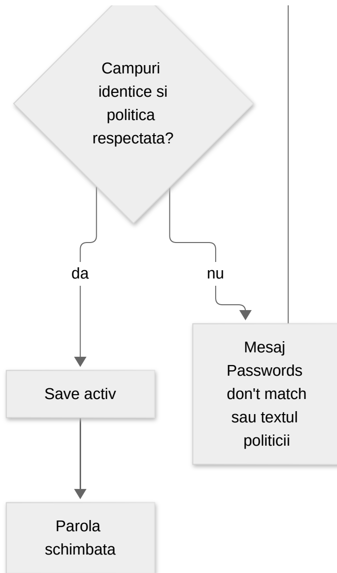
Figura 2: Desfășurarea dialogului „Change Password” – superutilizatorului nu i se cere parola anterioară.
