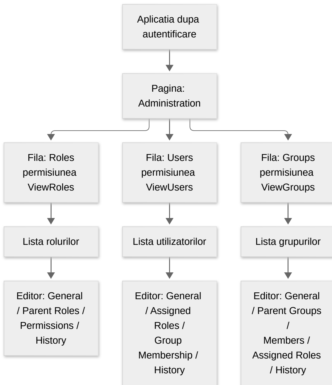
Figura 1: Structura paginilor interfeței de administrare – trei file dependente de permisiuni, fiecare cu o listă și un editor cu mai multe pagini.
