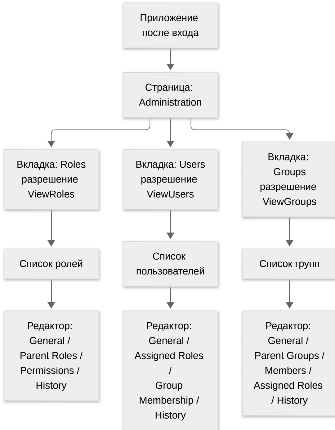
Рисунок 1: Структура страниц интерфейса администрирования — три зависящие от разрешений вкладки, каждая со списком и многостраничным редактором.
