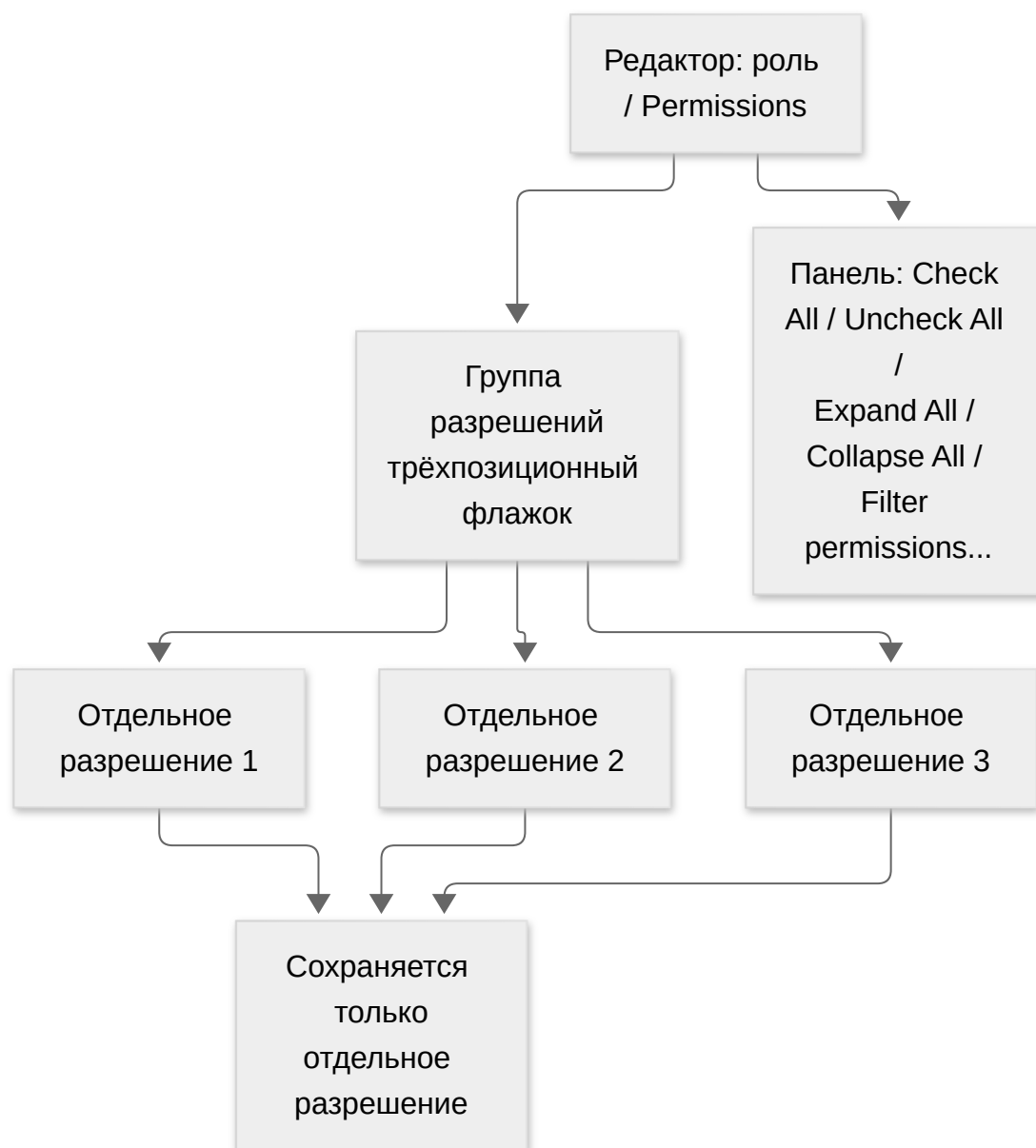
Рисунок 3: Строение выбора разрешений в редакторе ролей — группы служат для обзора, сохраняются отдельные разрешения.
