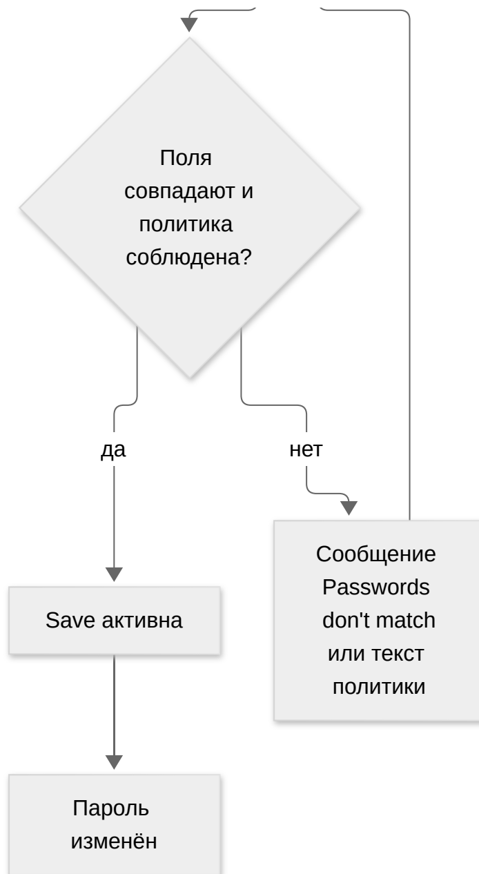
Рисунок 2: Ход диалога «Change Password» — у суперпользователя прежний пароль не запрашивается.
