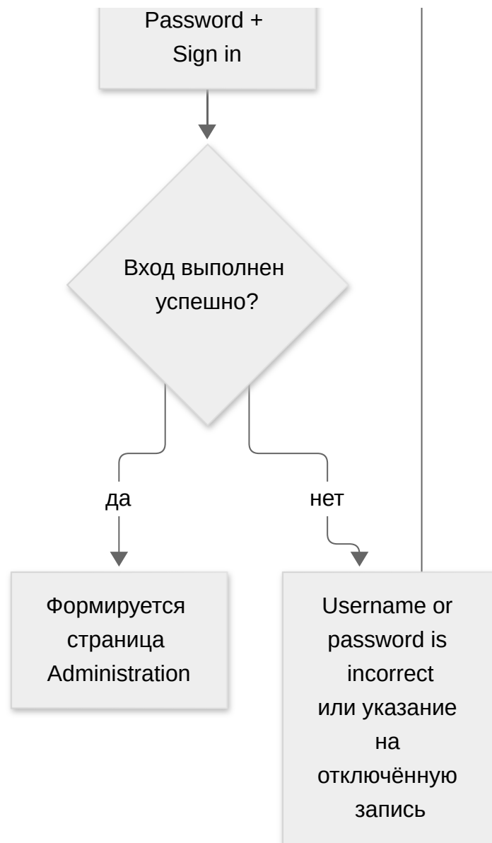
Рисунок 5: Путь от первого запуска через вход к странице администрирования.
