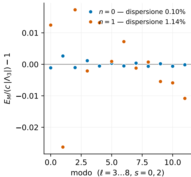
(b) residuo attorno alla costante
