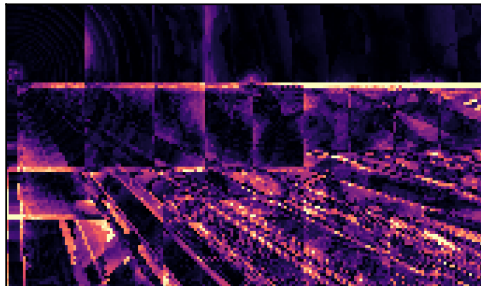
(d) Direct RF absolute error
