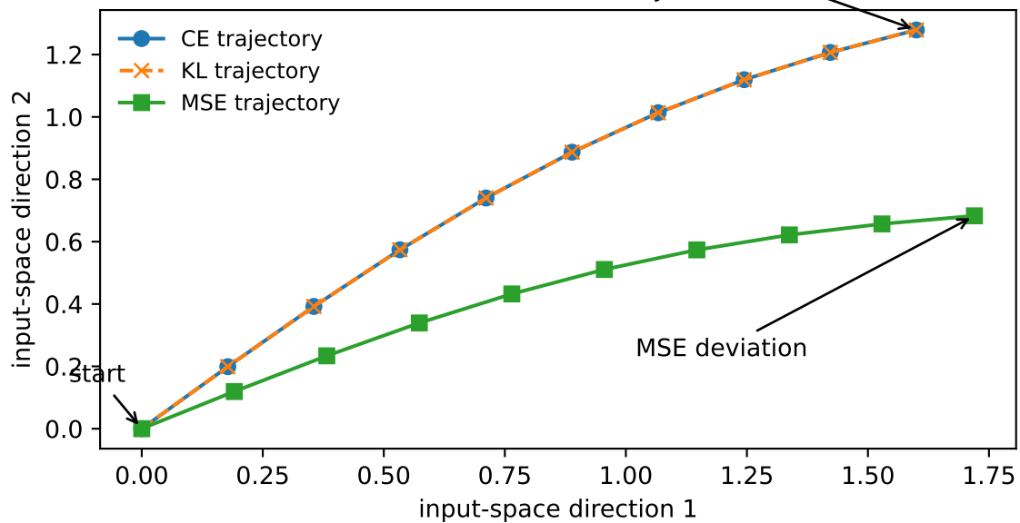
(d) Identical CE/KL trajectories
