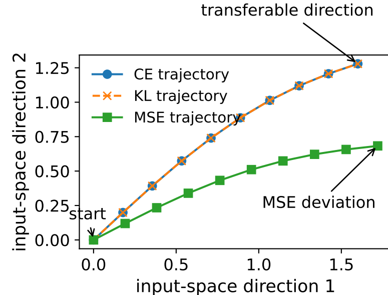
(d) Identical CE/KL trajectories
