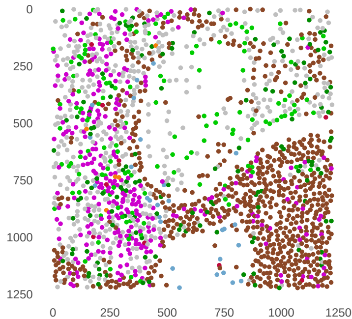
mIF sample 10071582 ROI 007
