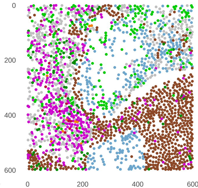
IMC sample 10071582 ROI 007
