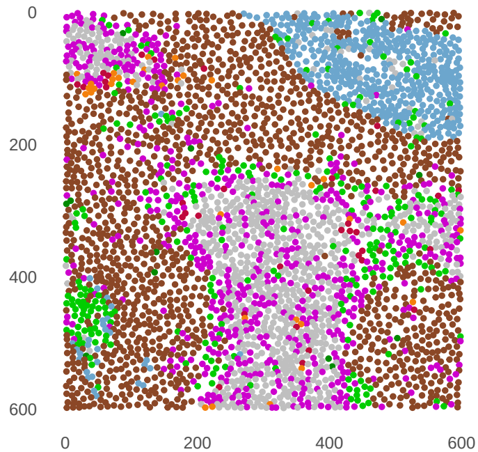
IMC sample 10068868 ROI 005
