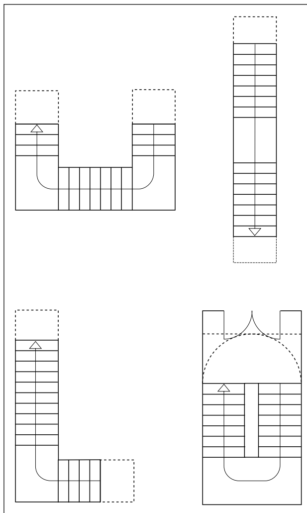
Abbildung 409-1: Fluchtwege
