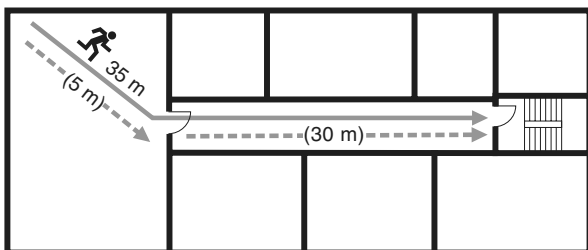
Treppenanlage mit langem Korridor
