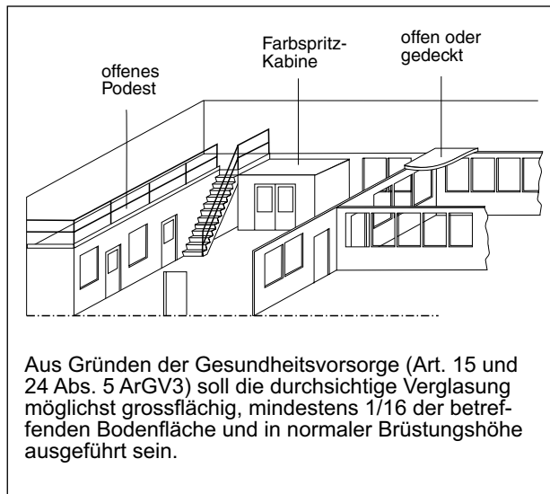
Abbildung 408-8: Raumeinbauten
