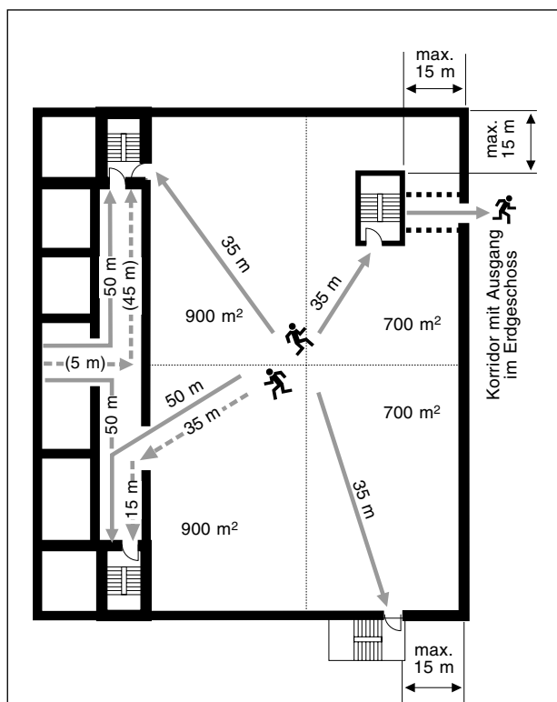
Abbildung 408-6: Beispiel für Geschosse mit vier Treppenanlagen
