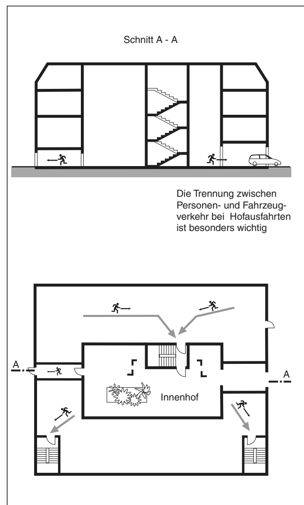
Abbildung 408-7: Beispiel für Gebäude mit Innenhof
