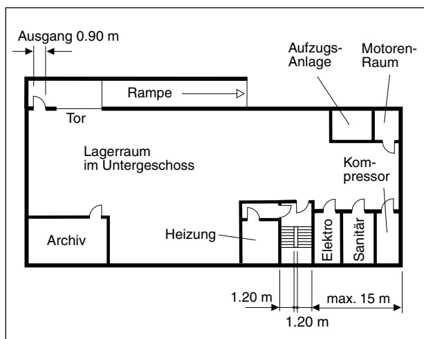
Abbildung 408-9: Betriebsbezogene Anlagenräume
