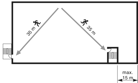
Zwei Treppenanlagen ohne Korridor
