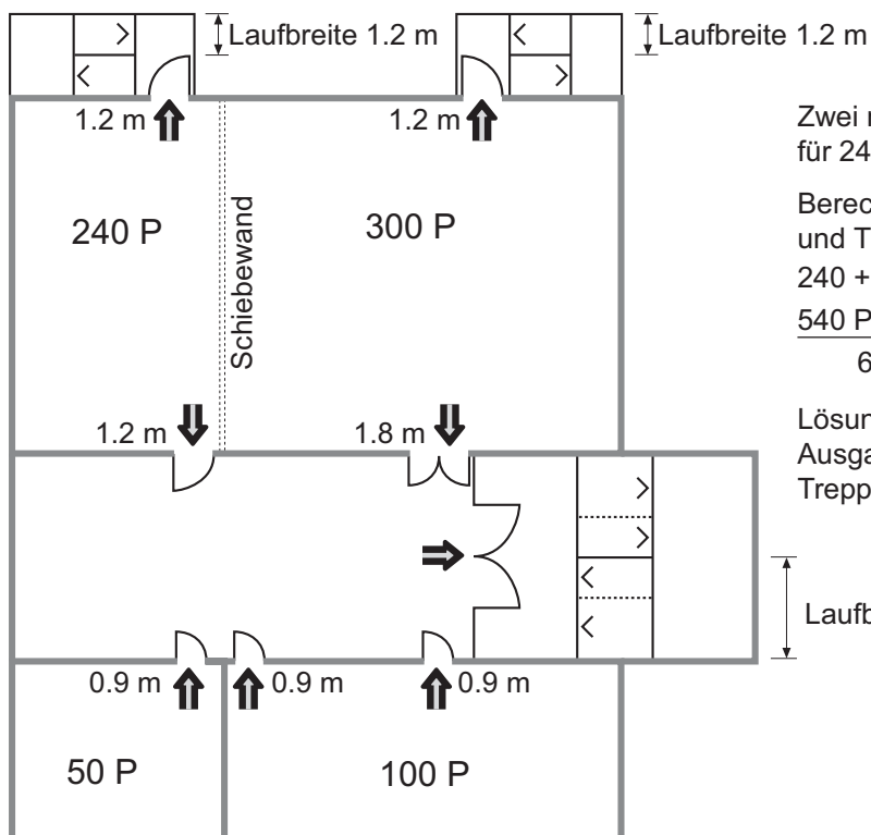
Obergeschoss
