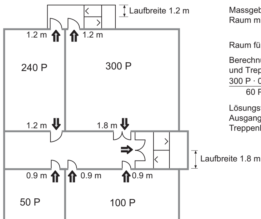
Obergeschoss
