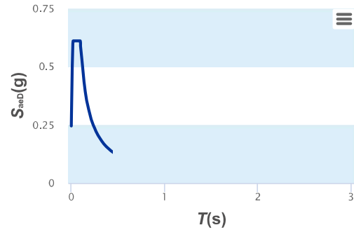
Düşey Elastik Tasarım Spektrumu
