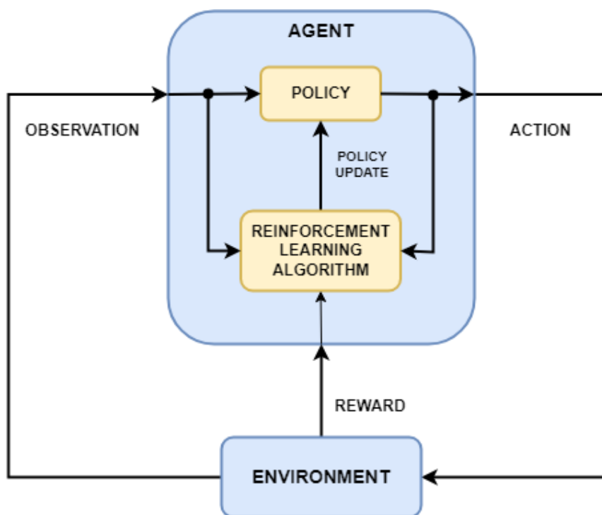
شکل (۱-۲) چارچوب کلی یادگیری تقویتی [۱۴].
