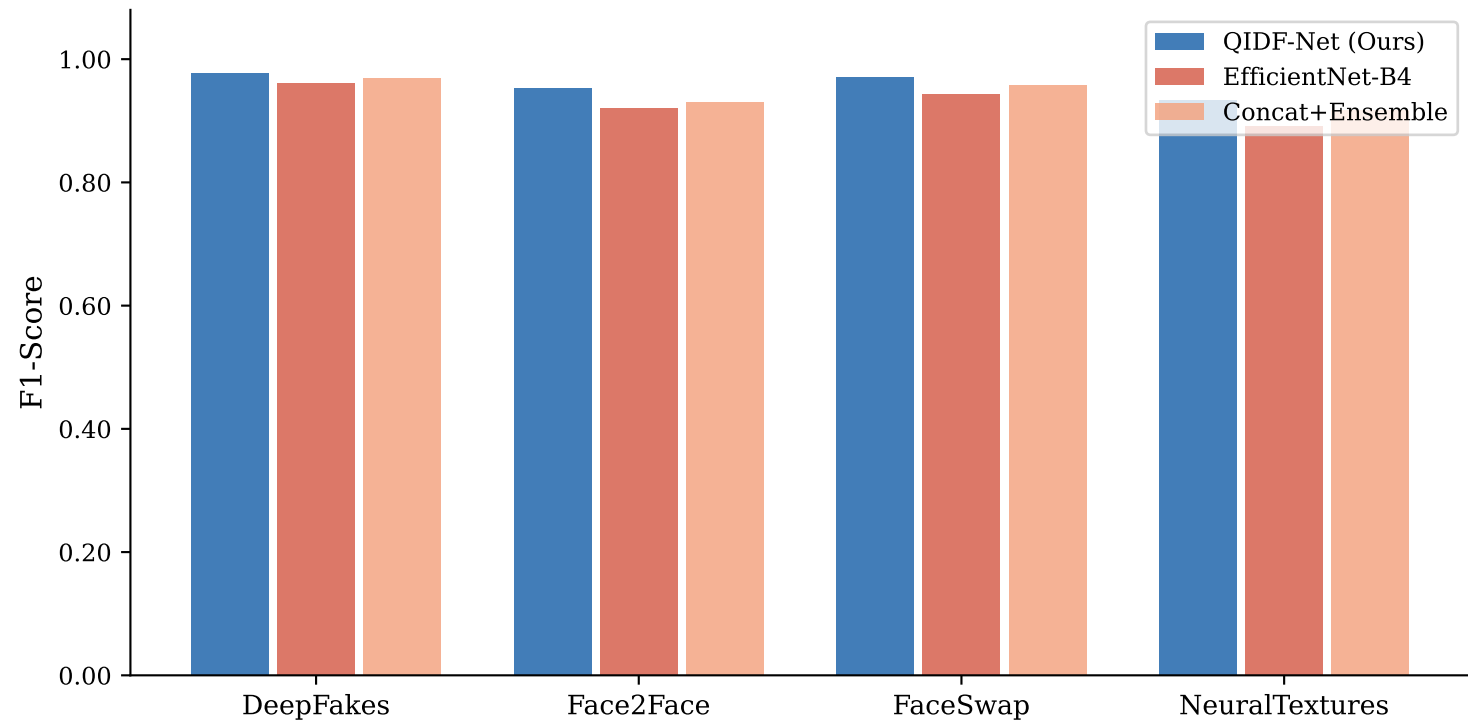
Per-Manipulation-Type F1 Score
