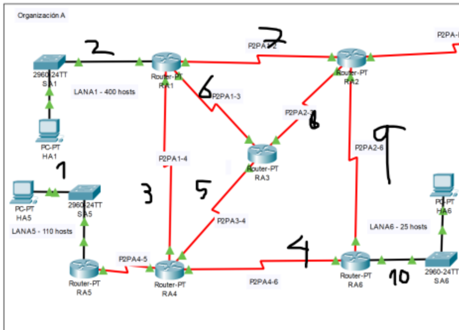
Figura 1. Topología de red de la organización A
