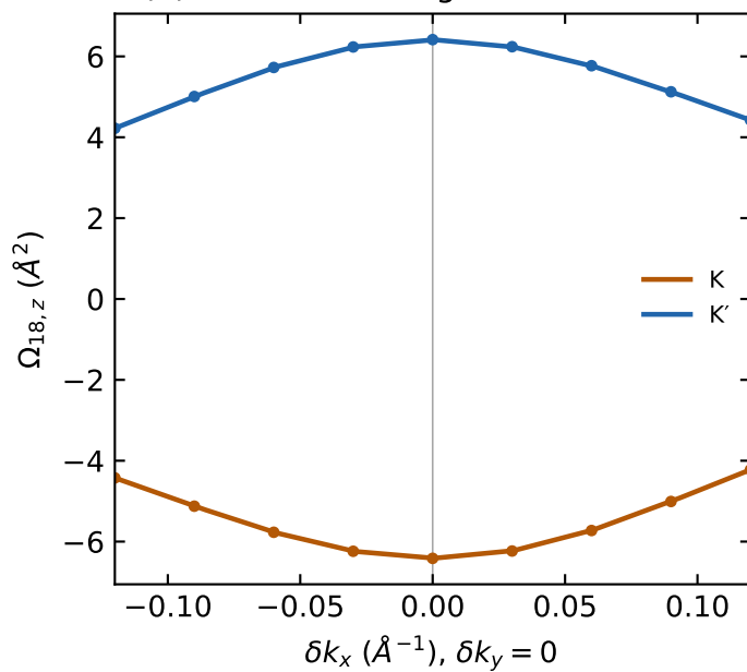
(d) Curvature along the dashed cuts
