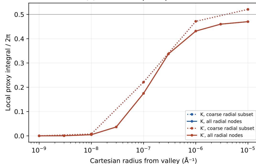
(d) Local native point quadrature
