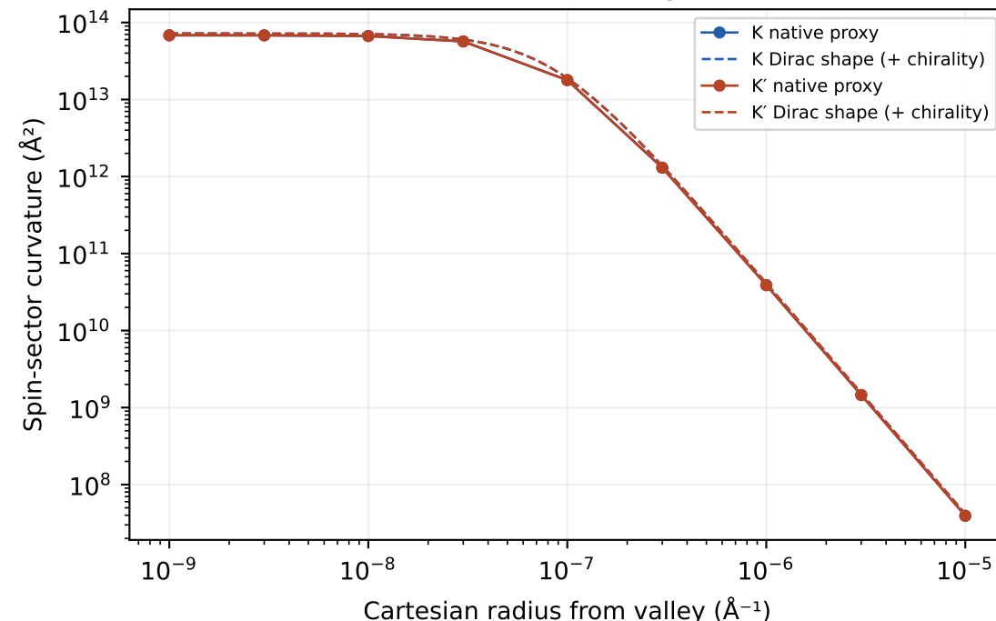
(d) Local native point quadrature
