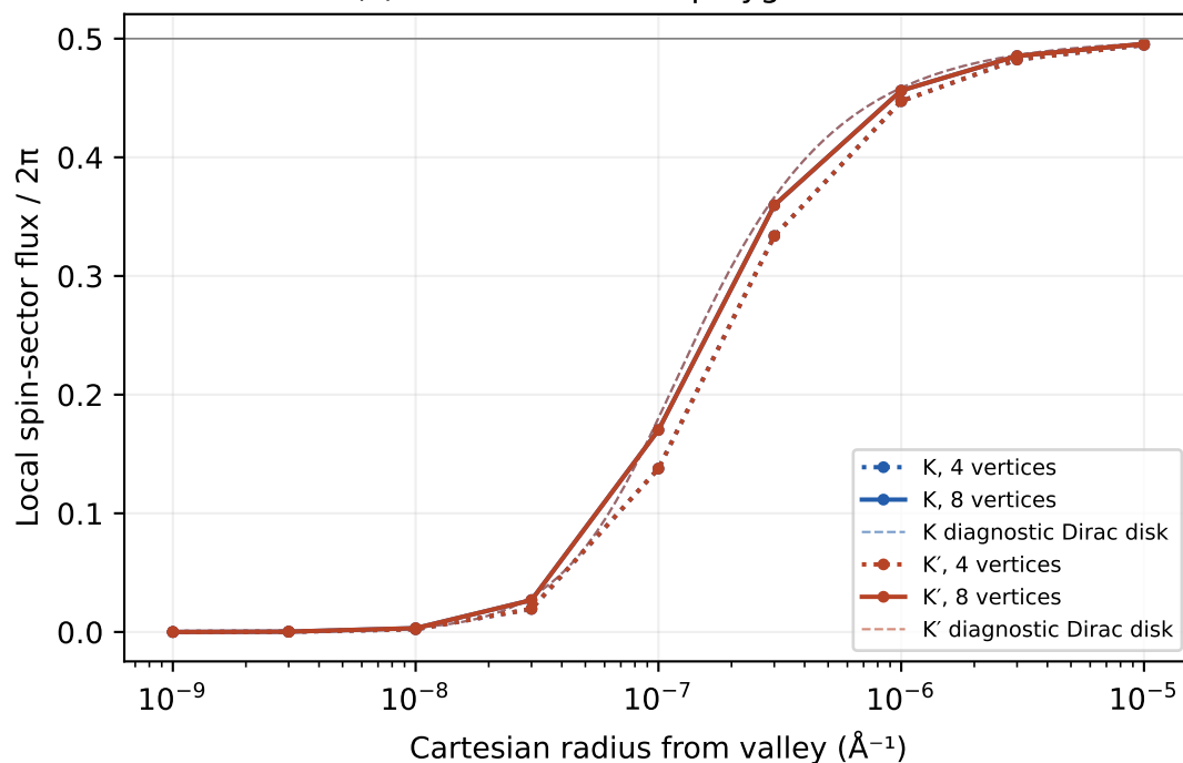
(c) Actual WAVECAR polygon flux / 2\pi
