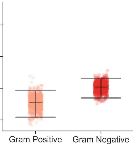
ROC-AUC
