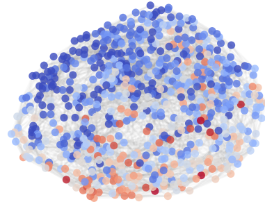
CNS Rate
