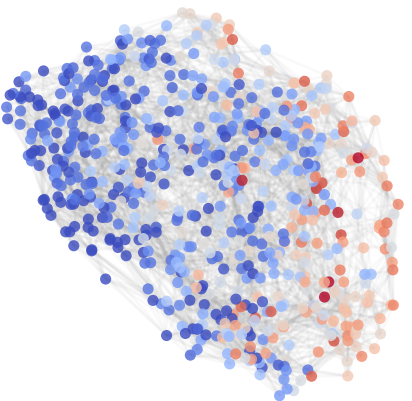
CNS Rate
