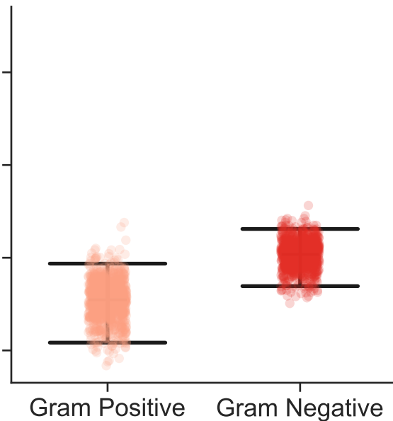
ROC-AUC
