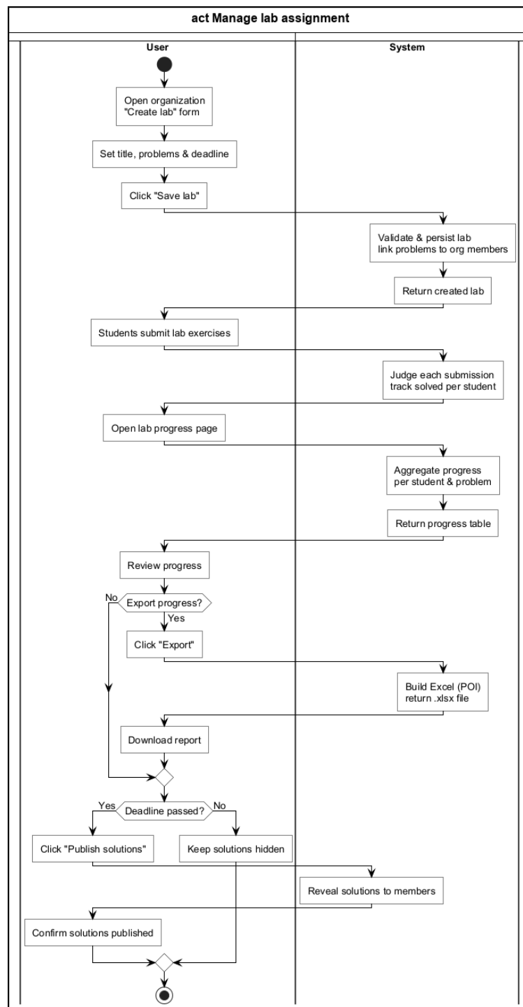
Hình 3.12: Sơ đồ hoạt động cho Use Case Quản lý bài thực hành
