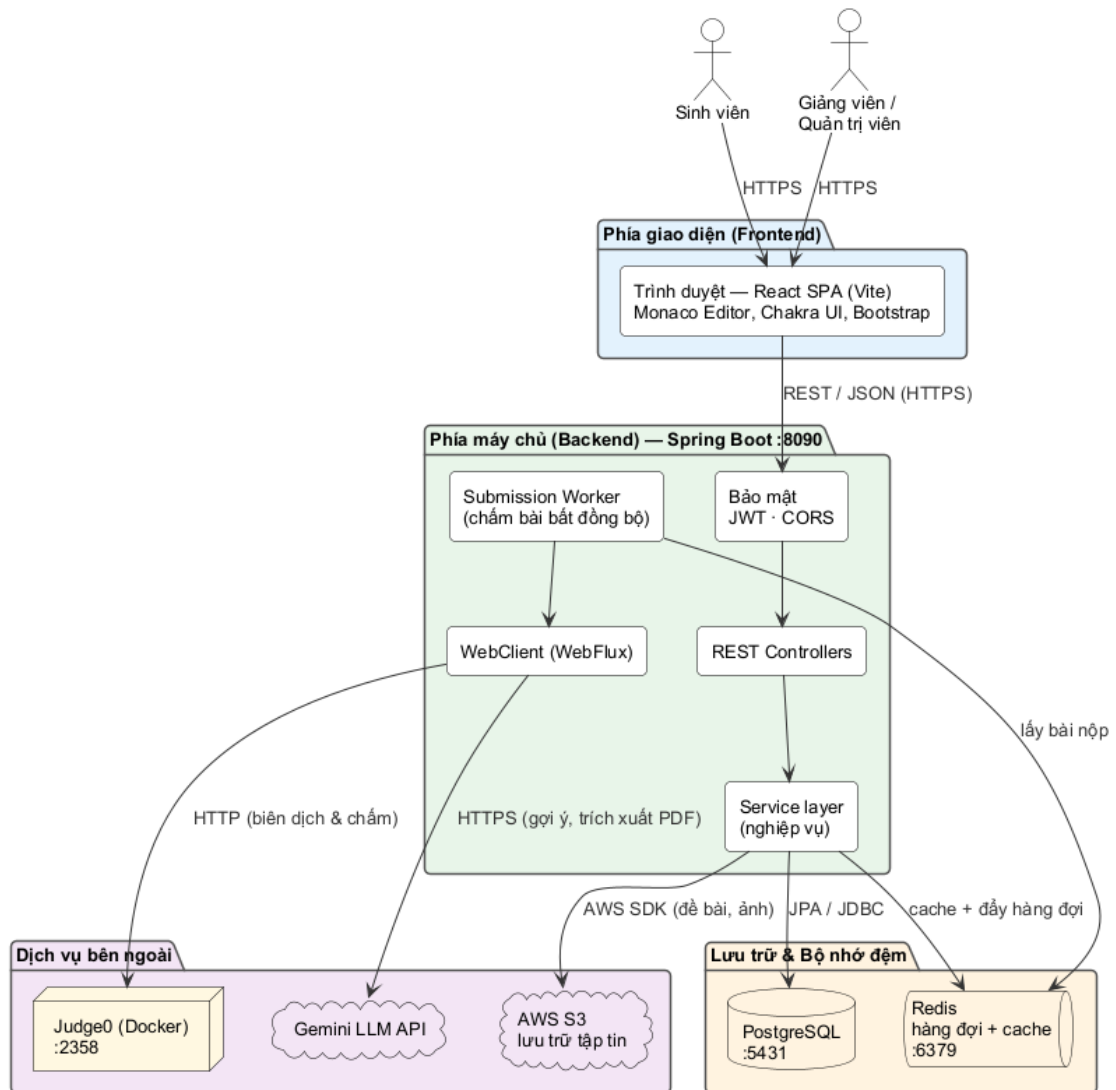
Hình 4.1: Kiến trúc tổng quan của hệ thống TDTUOJ
