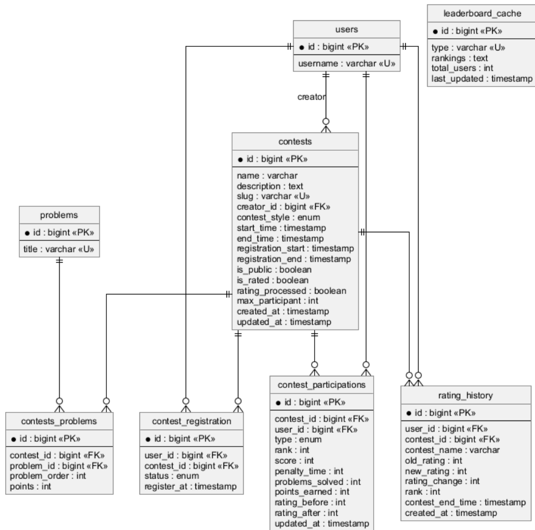
Hình 4.6: Phân mảnh ERD – Cuộc thi
