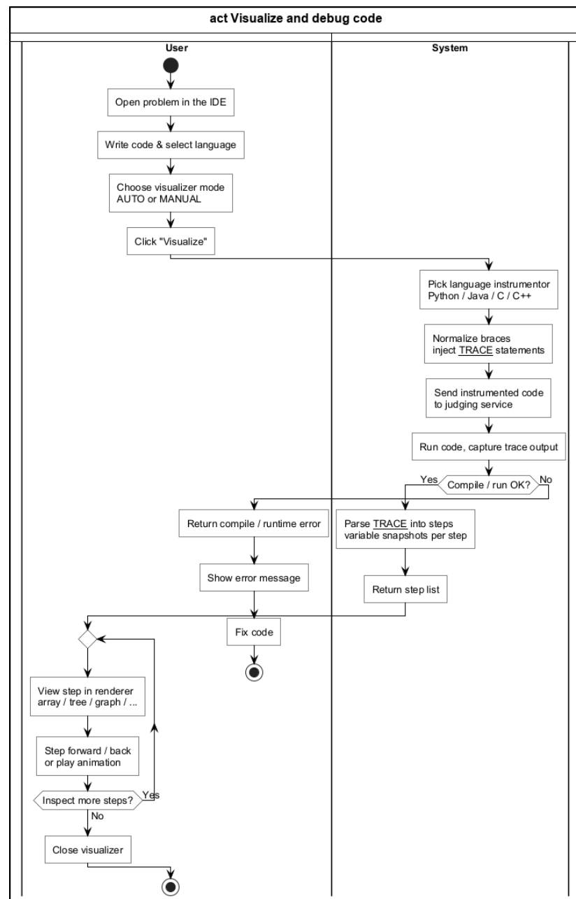
Hình 3.6: Sơ đồ hoạt động cho Use Case Trực quan hóa và gỡ lỗi mã nguồn
