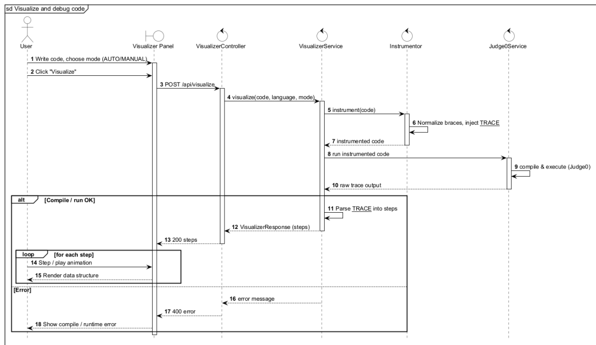
Hình 3.7: Sơ đồ tuần tự cho Use Case Trực quan hóa và gỡ lỗi mã nguồn
