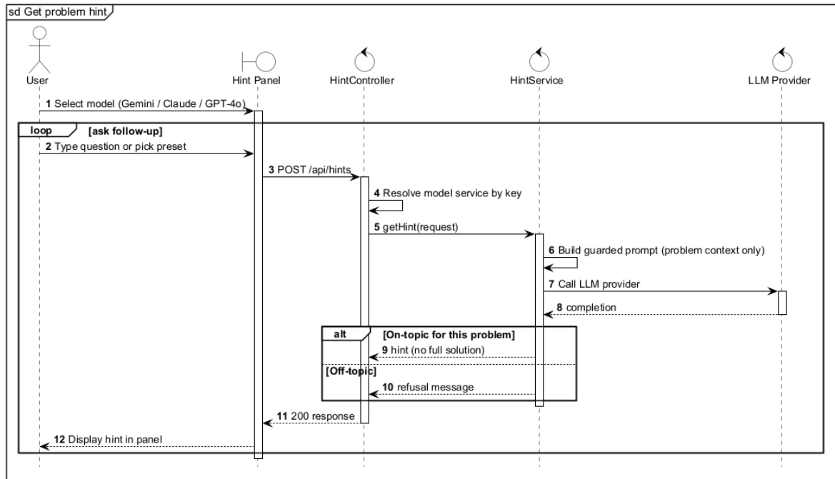
Hình 3.11: Sơ đồ tuần tự cho Use Case Gợi ý học tập bằng LLM
