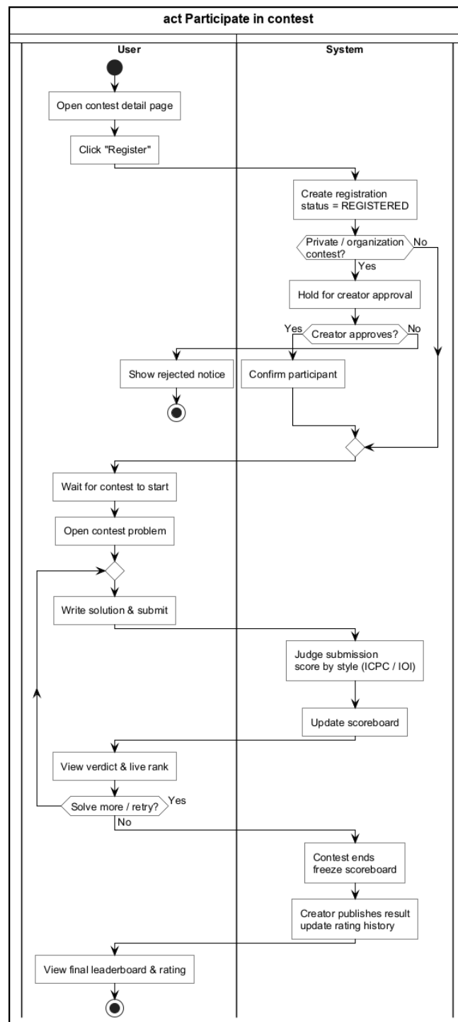
Hình 3.8: Sơ đồ hoạt động cho Use Case Tham gia cuộc thi
