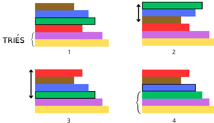
Figure 1: Une étape de tri : on fait remonter l'élément à trier en haut, puis on le redescend à la bonne position
