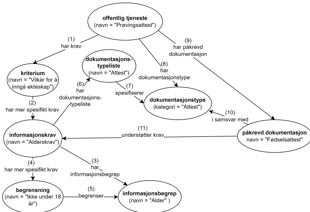
Figur 13. Eksempel - beskrivelse av «alderskrav» til tjenesten «prøvingsattest».
