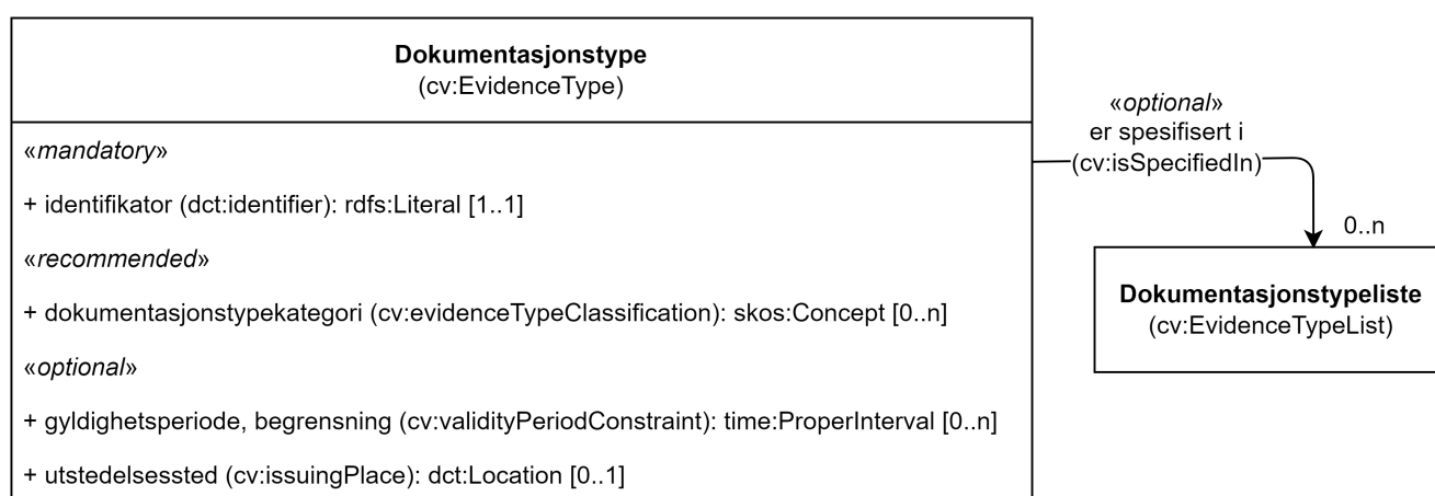
Figur 4. Klassen Dokumentasjonstype (cv:EvidenceType) og klassen den refererer til.
