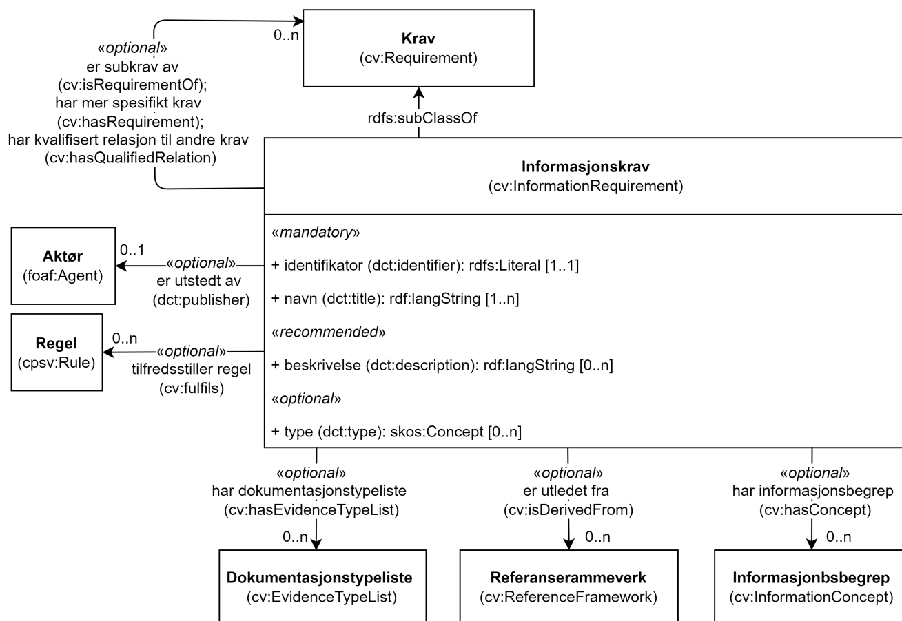
Figur 7. Klassen Informasjonskrav (cv:InformationRequirement) og klassene den refererer til.
