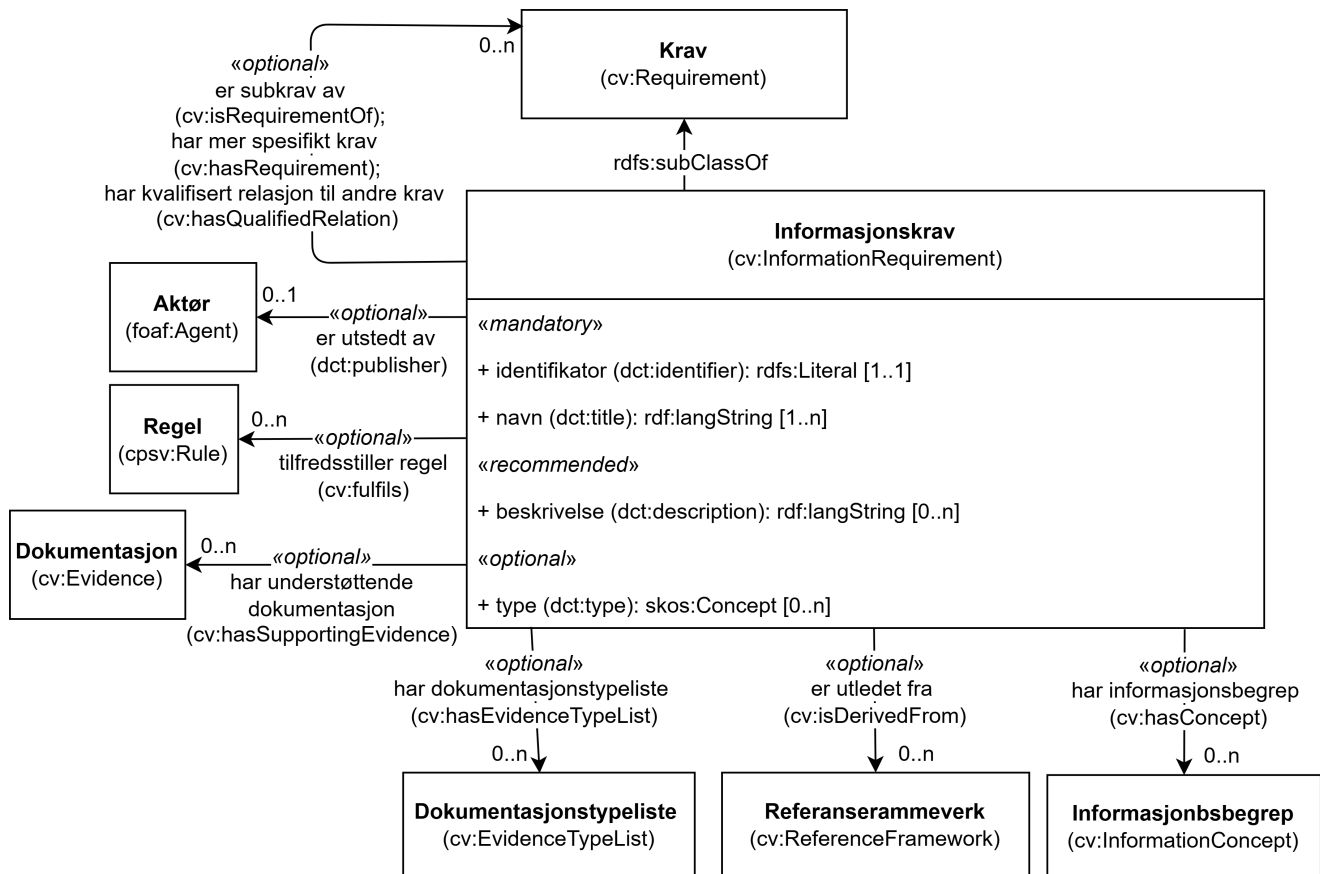
Figur 8. Klassen Informasjonskrav (cv:InformationRequirement) og klassene den refererer til.
