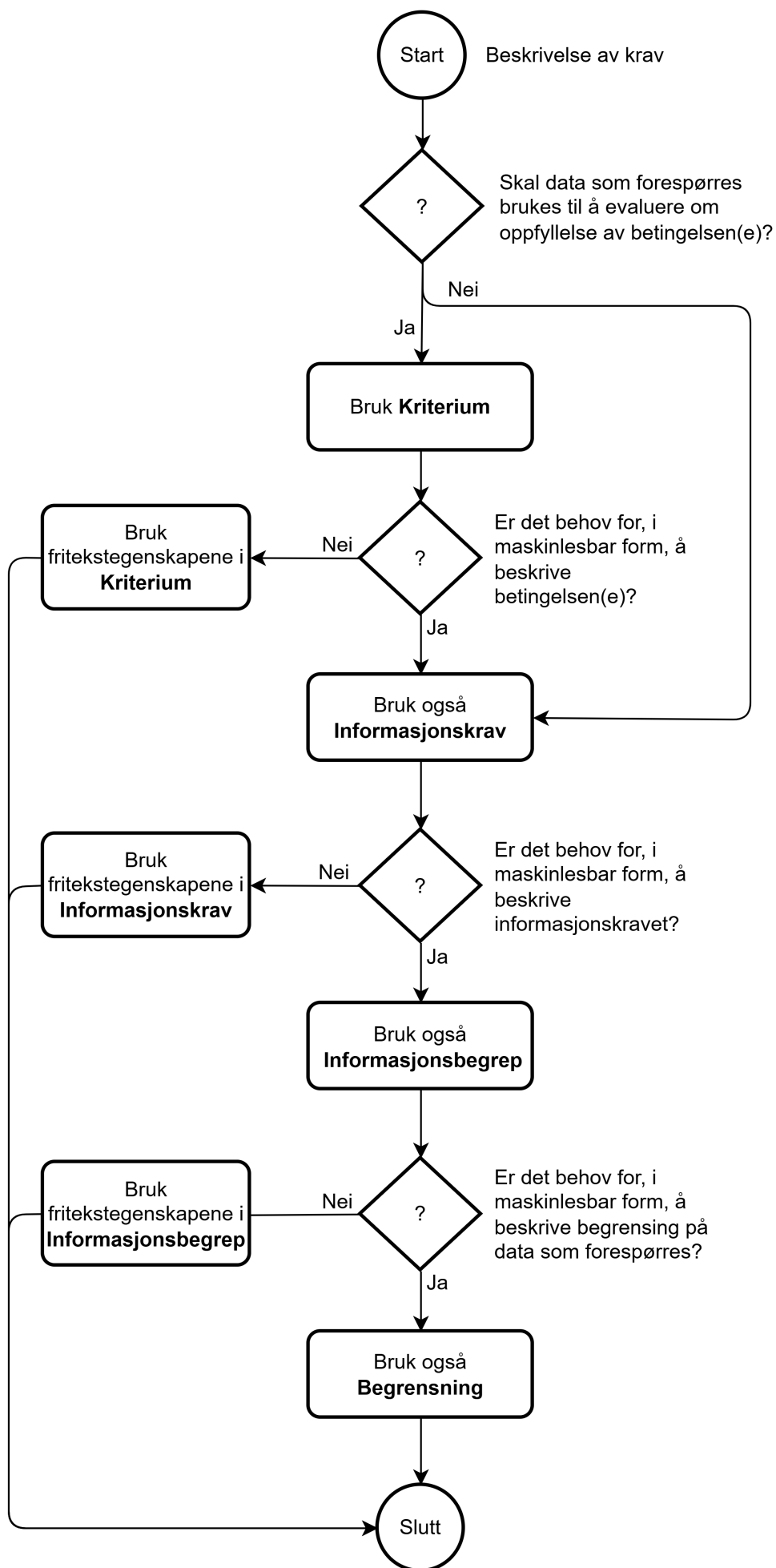
Figur 14. Flytskjema for når Kriterium, Informasjonskrav eller Begrensning bør brukes.
