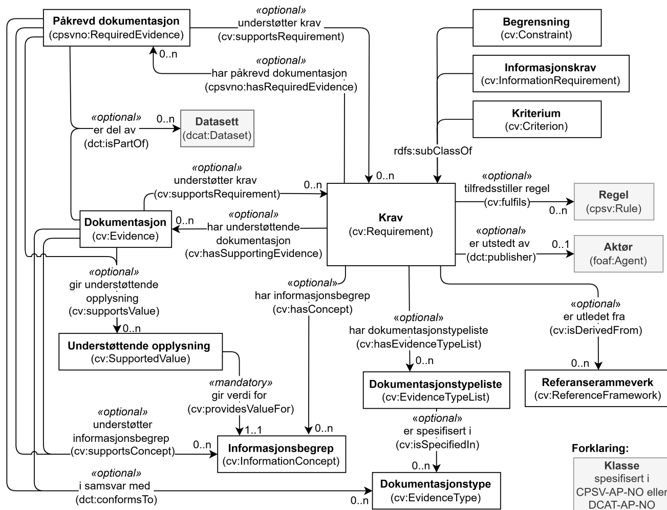
Figur 2. Klassene i CCCEV-AP-NO.
