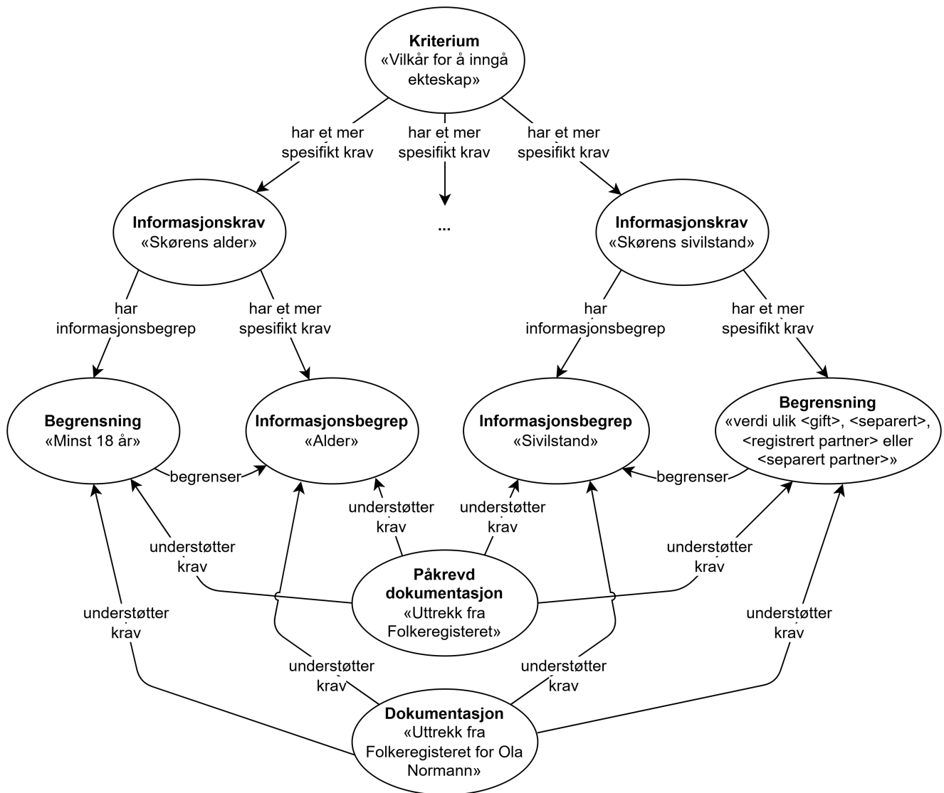
Figur 15. Eksempel - beskrivelse av «vilkår for å inngå ekteskap».
