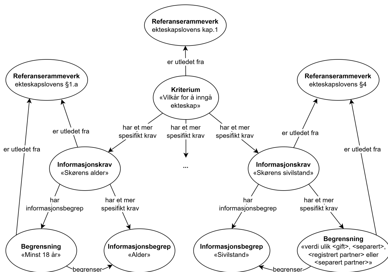
Figur 16. Eksempel på å knytte dokumentasjonskrav til lovgivning.
