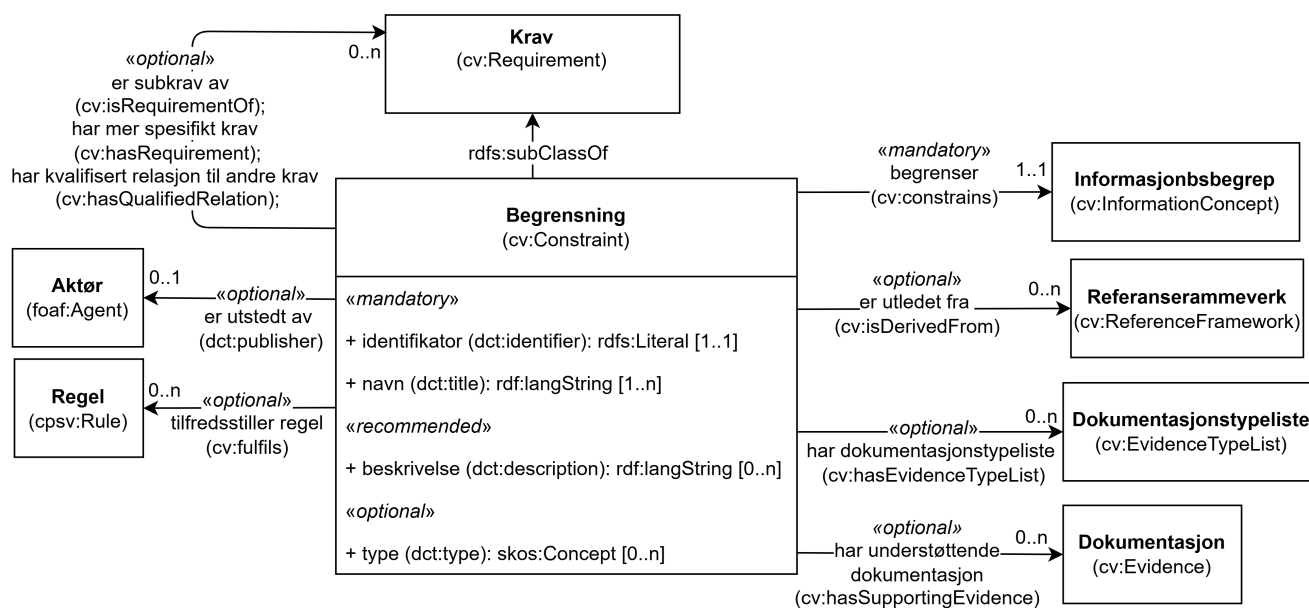
Figur 3. Klassen Begrensning (cv:Constraint) og klassene den refererer til.
