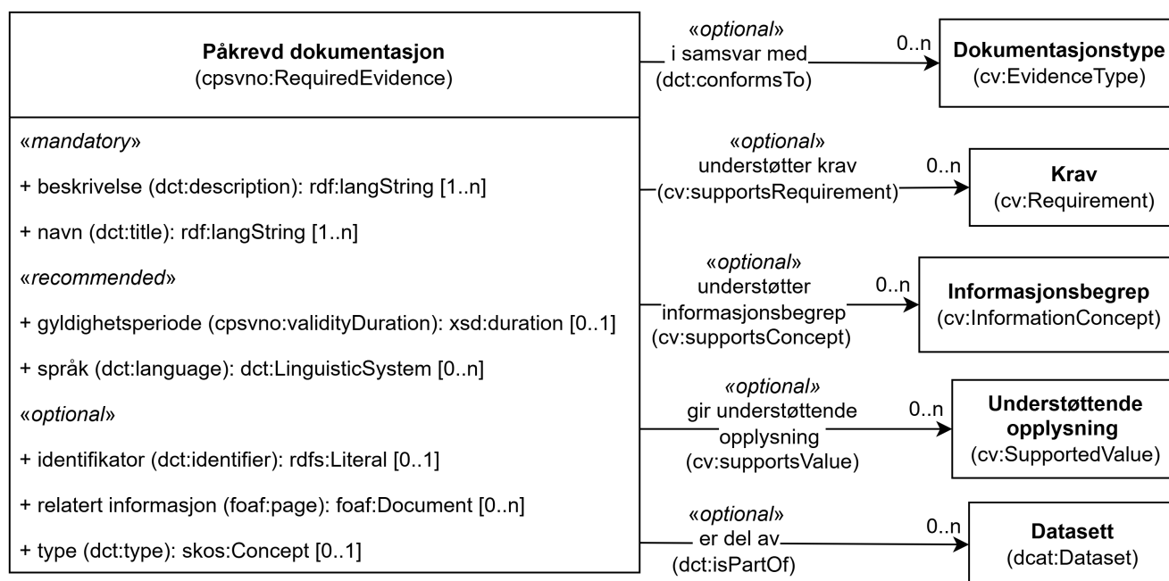
Figur 11. Klassen Påkrevd dokumentasjon (cpsvno:RequiredEvidence) og klassene den refererer til.
