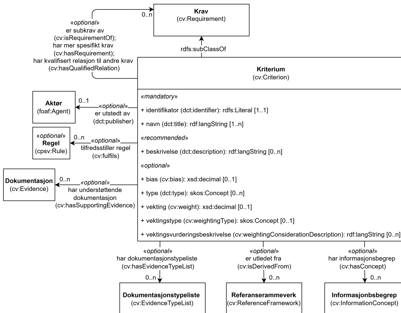
Figur 10. Klassen Kriterium (cv:Criterion) og klassene den refererer til.
