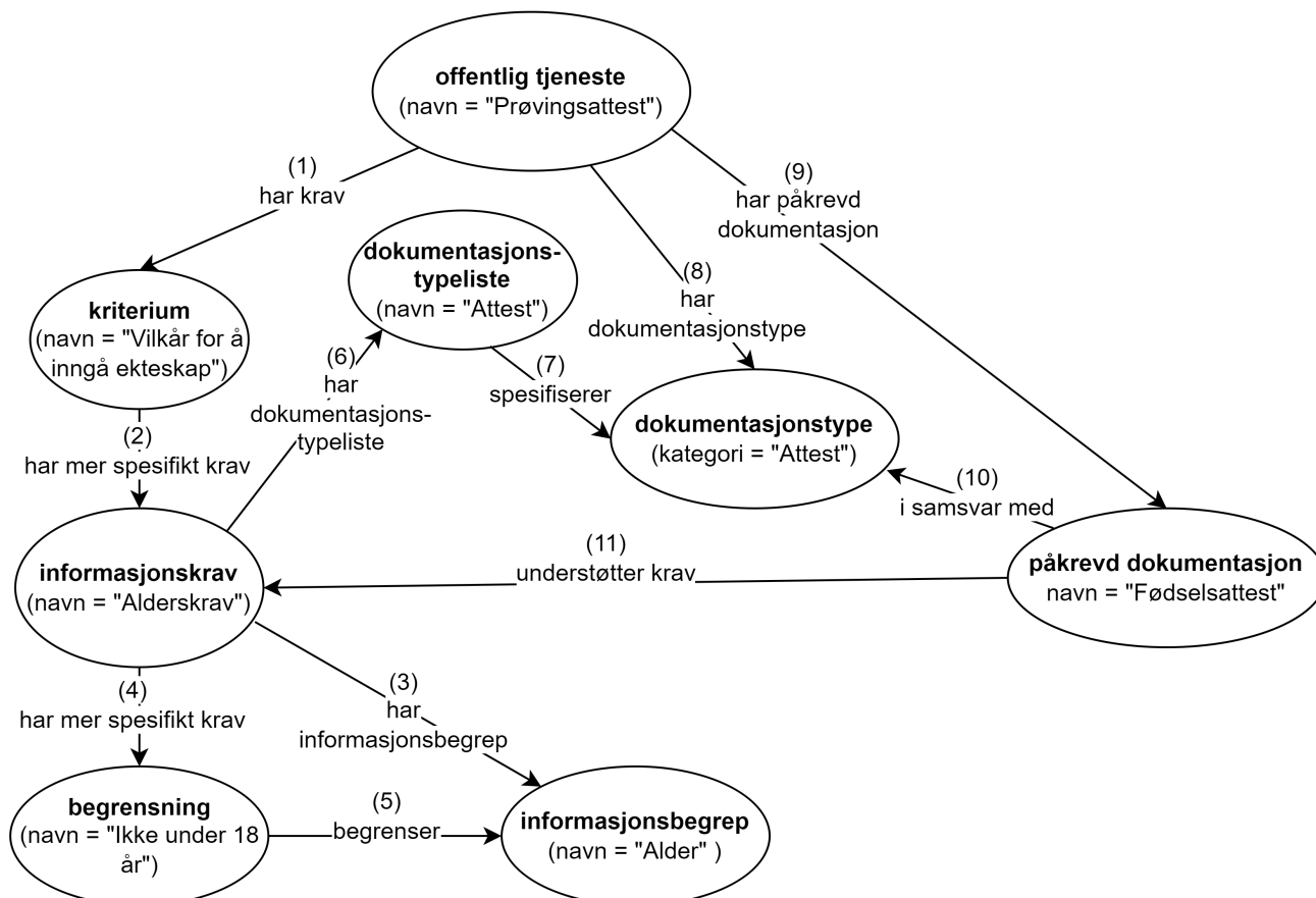
Figur 8. Eksempel - beskrivelse av «alderskrav» til tjenesten «prøvingsattest».
