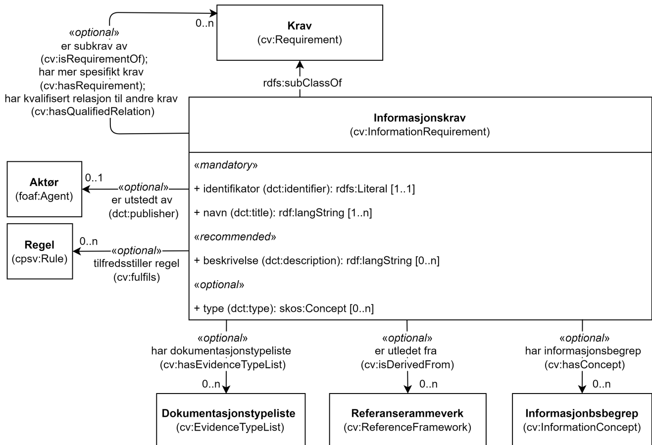
Figur 4. Klassen Informasjonskrav (cv:InformationRequirement) og klassene den refererer til.
