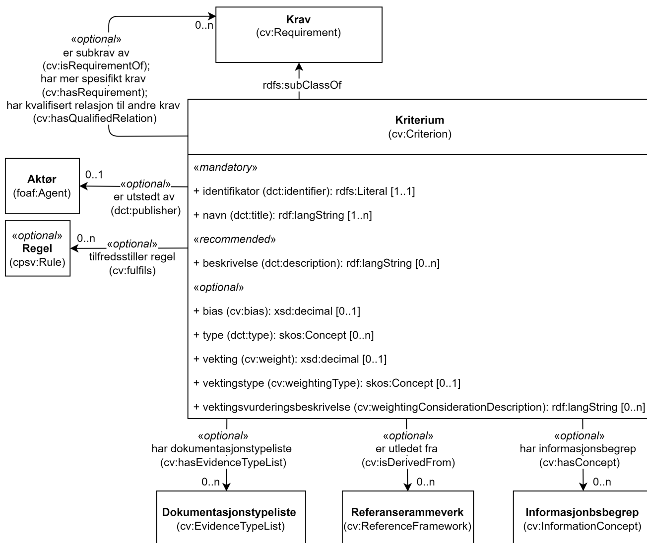
Figur 6. Klassen Kriterium (cv:Criterion) og klassene den refererer til.
