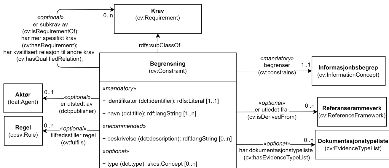
Figur 1. Klassen Begrensning (cv:Constraint) og klassene den refererer til.
