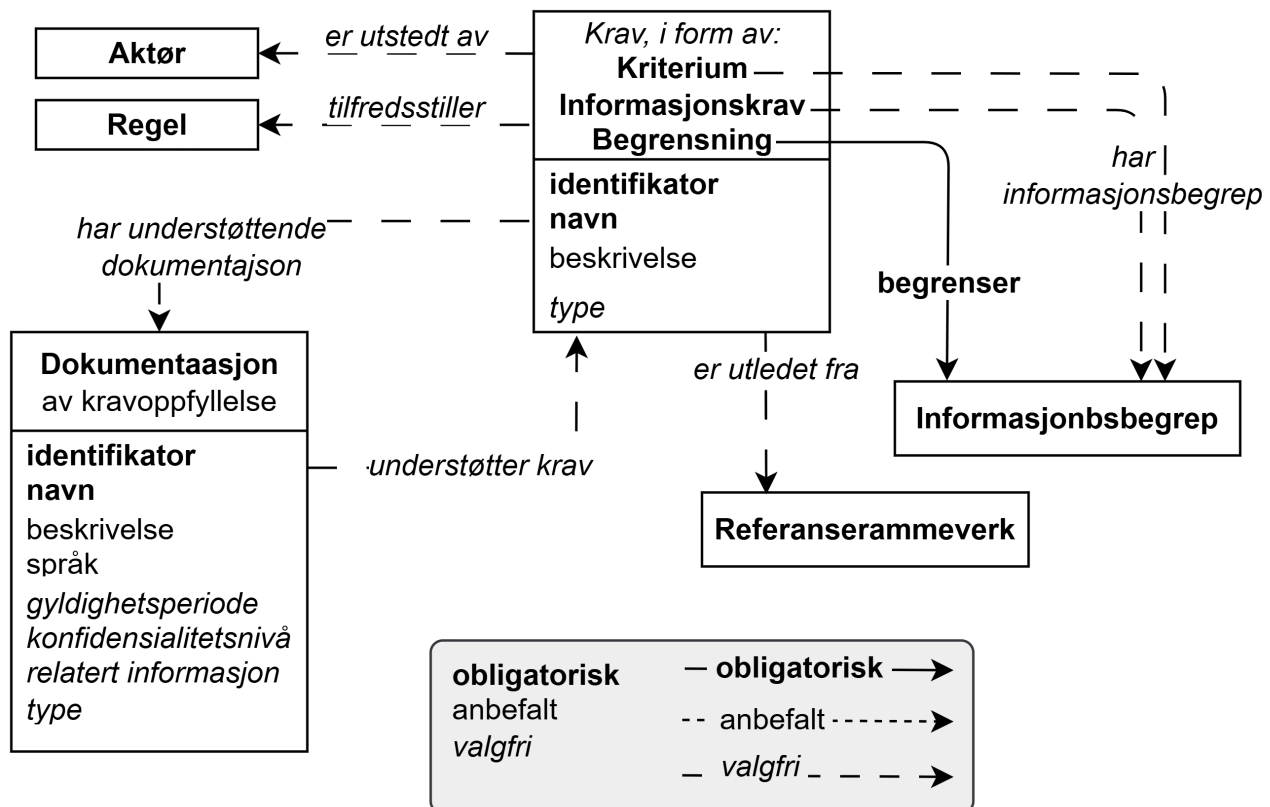
Figur 1. Forenklet fremstilling av noen av kravene i CCCEV-AP-NO
