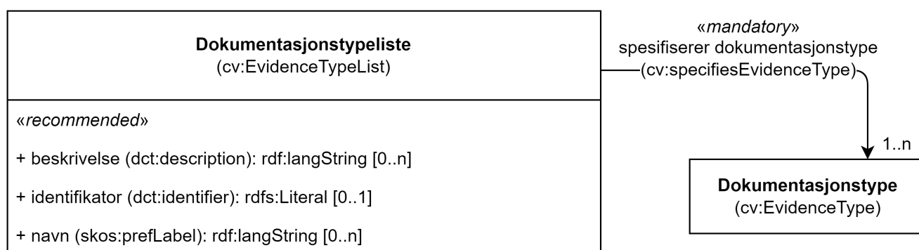
Figur 3. Klassen Dokumentasjonstypeliste (cv:EvidenceTypeList) og klassen den refererer til.
