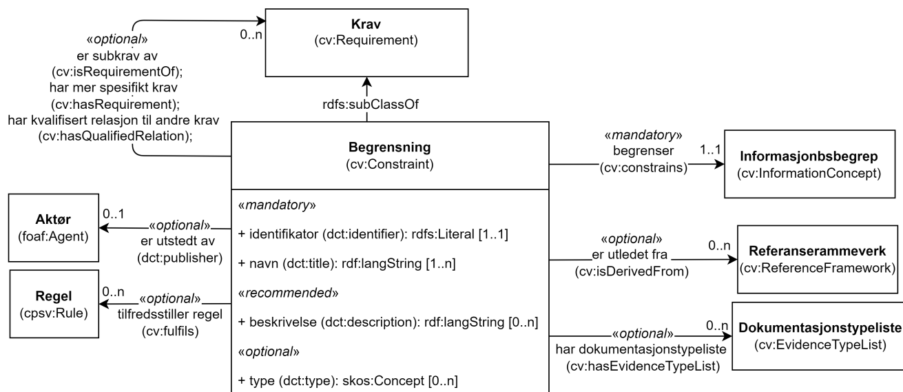
Figur 2. Klassen Begrensning (cv:Constraint) og klassene den refererer til.
