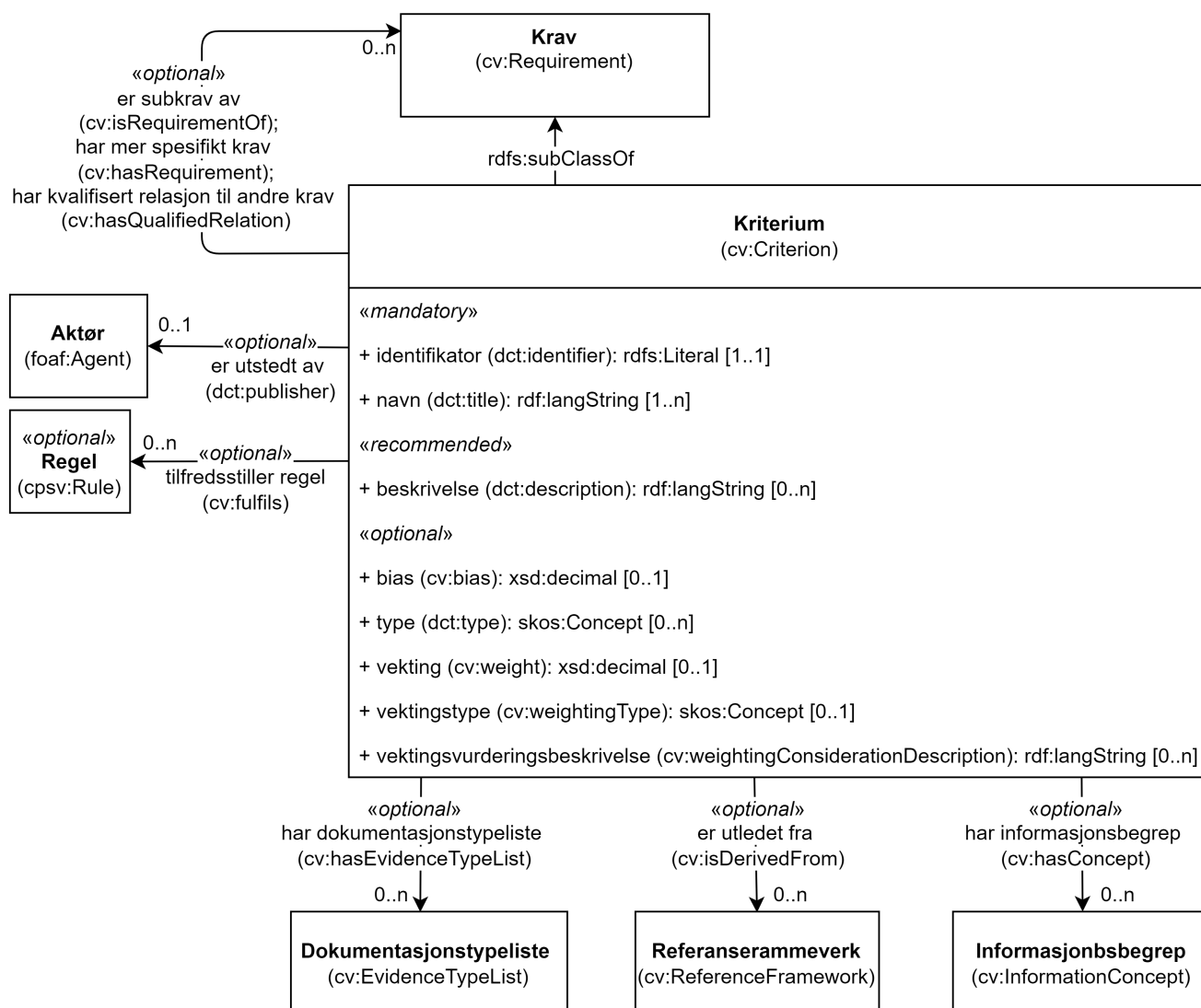
Figur 7. Klassen Kriterium (cv:Criterion) og klassene den refererer til.
