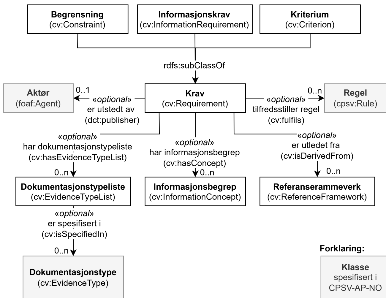
Figur 1. Klassene i CCCEV-AP-NO.
