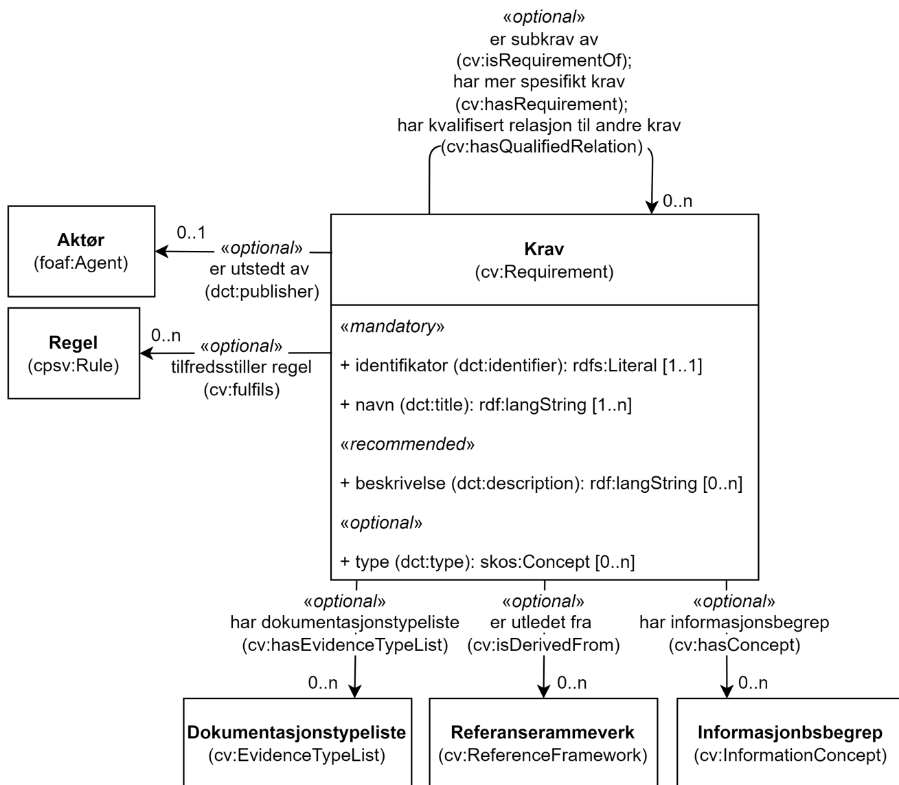
Figur 6. Klassen Krav (cv:Requirement) og klassene den refererer til.
