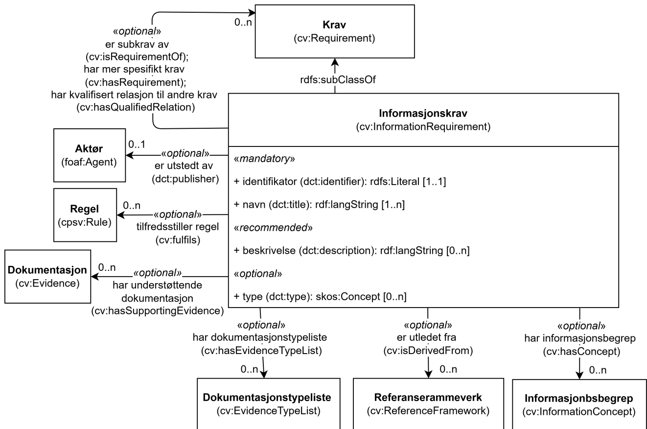
Figur 7. Klassen Informasjonskrav (cv:InformationRequirement) og klassene den refererer til.
