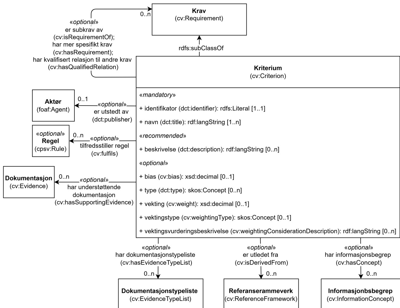
Figur 9. Klassen Kriterium (cv:Criterion) og klassene den refererer til.
