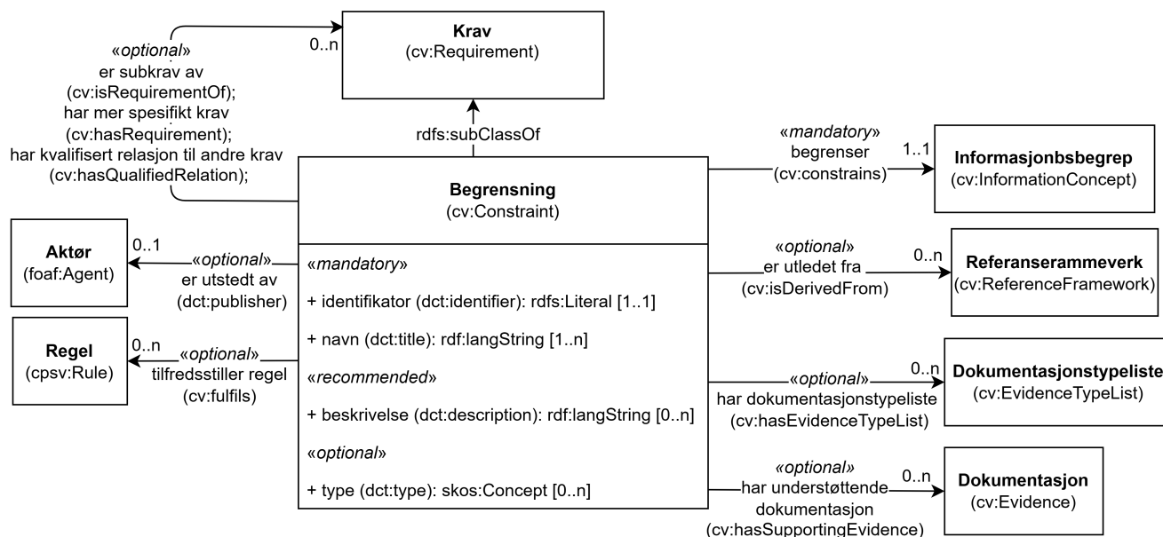
Figur 2. Klassen Begrensning (cv:Constraint) og klassene den refererer til.
