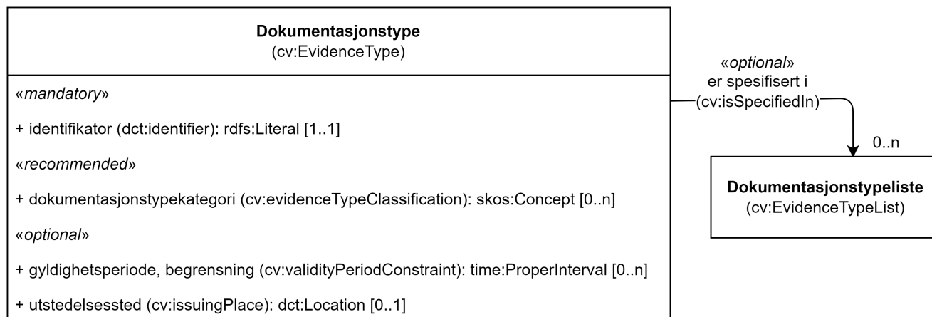
Figur 4. Klassen Dokumentasjonstype (cv:EvidenceType) og klassen den refererer til.
