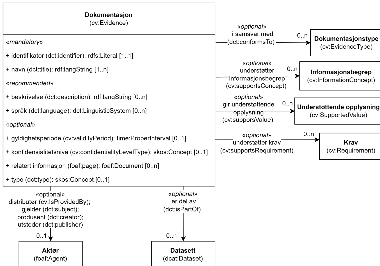
Figur 3. Klassen Dokumentasjon (cv:Evidence) og klassene den refererer til.
