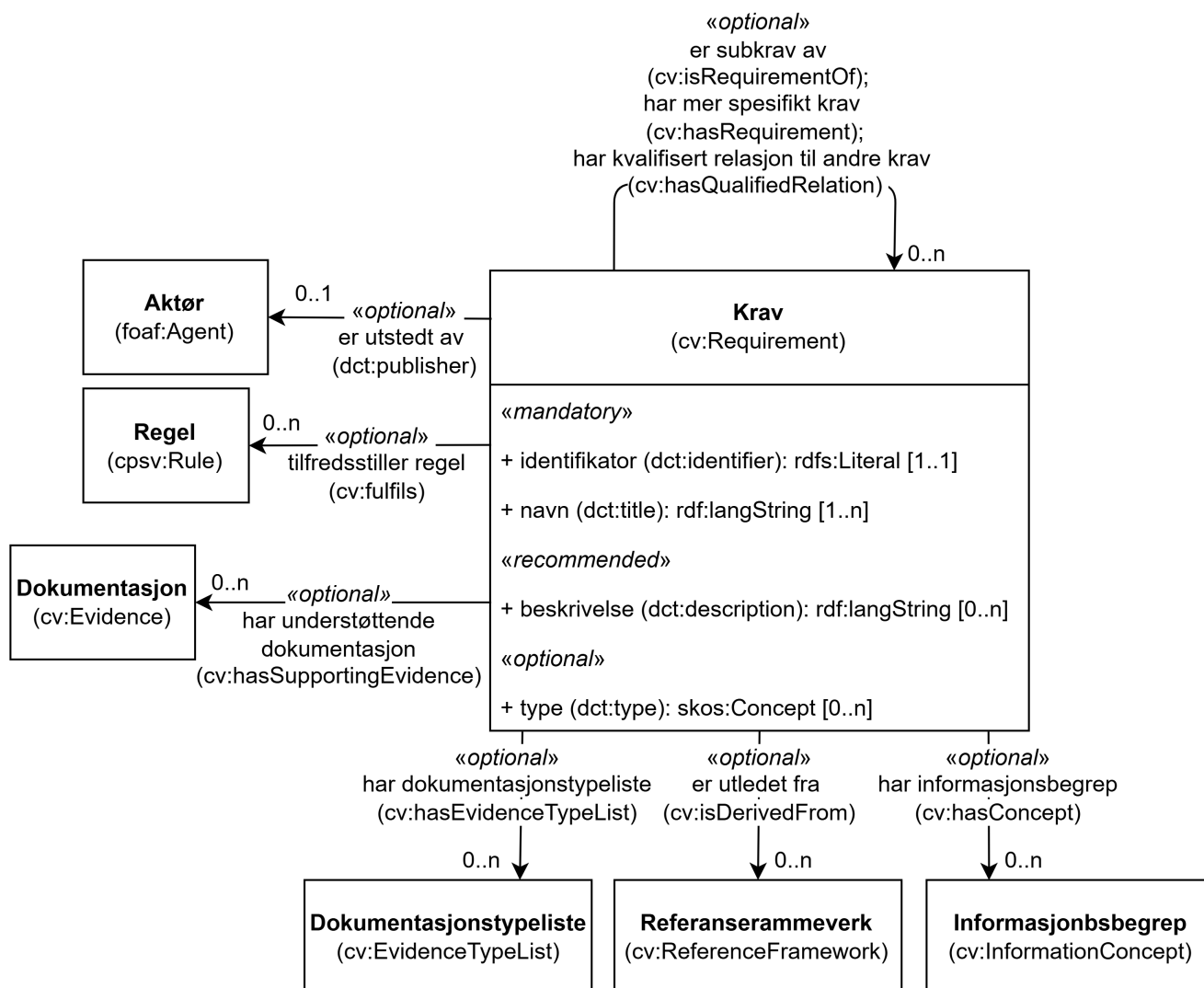
Figur 8. Klassen Krav (cv:Requirement) og klassene den refererer til.
