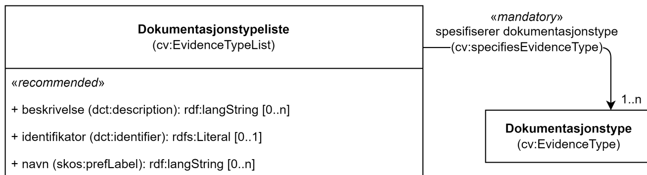
Figur 5. Klassen Dokumentasjonstypeliste (cv:EvidenceTypeList) og klassen den refererer til.
