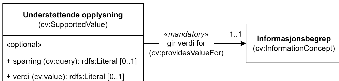
Figur 11. Klassen Understøttende opplysning (cv:SupportedValue) og klassen den refererer til.
