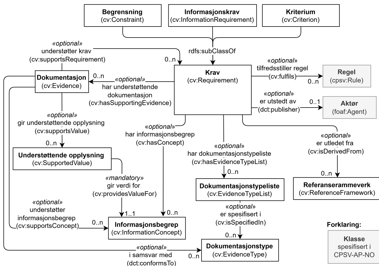
Figur 1. Klassene i CCCEV-AP-NO.
