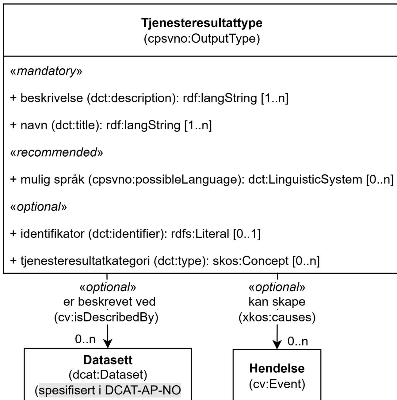
Figur 26. Klassen Tjenesteresultattype (cpsvno:OutputType) og klassene den refererer til.
