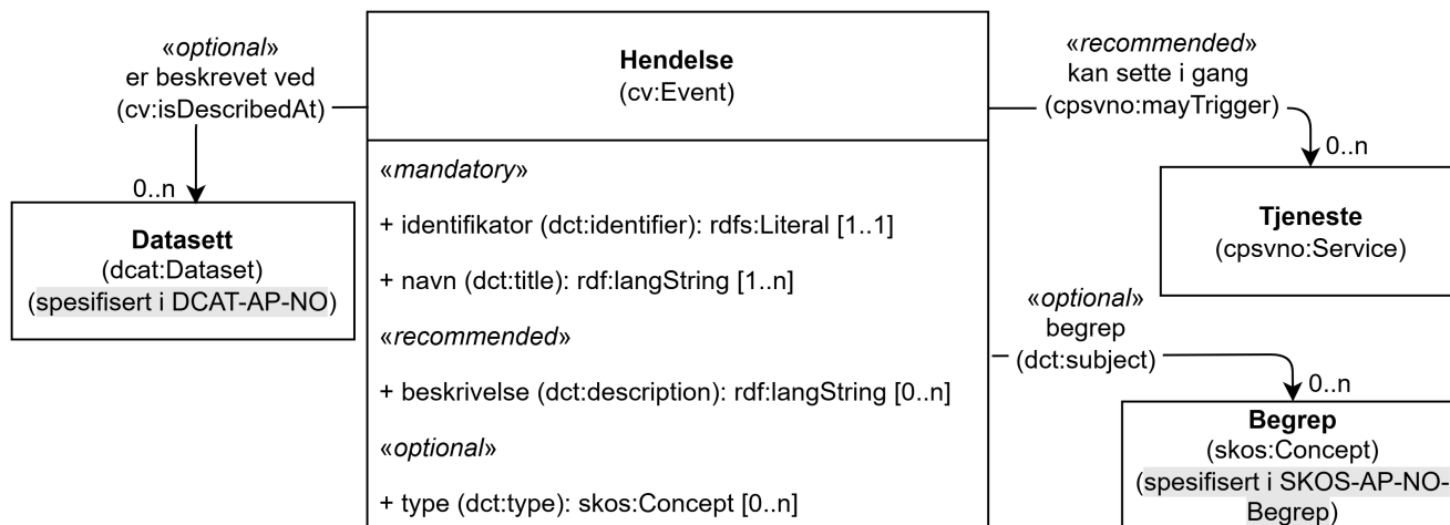
Figur 10. Klassen Hendelse (cv:Event) og klassene den refererer til.
