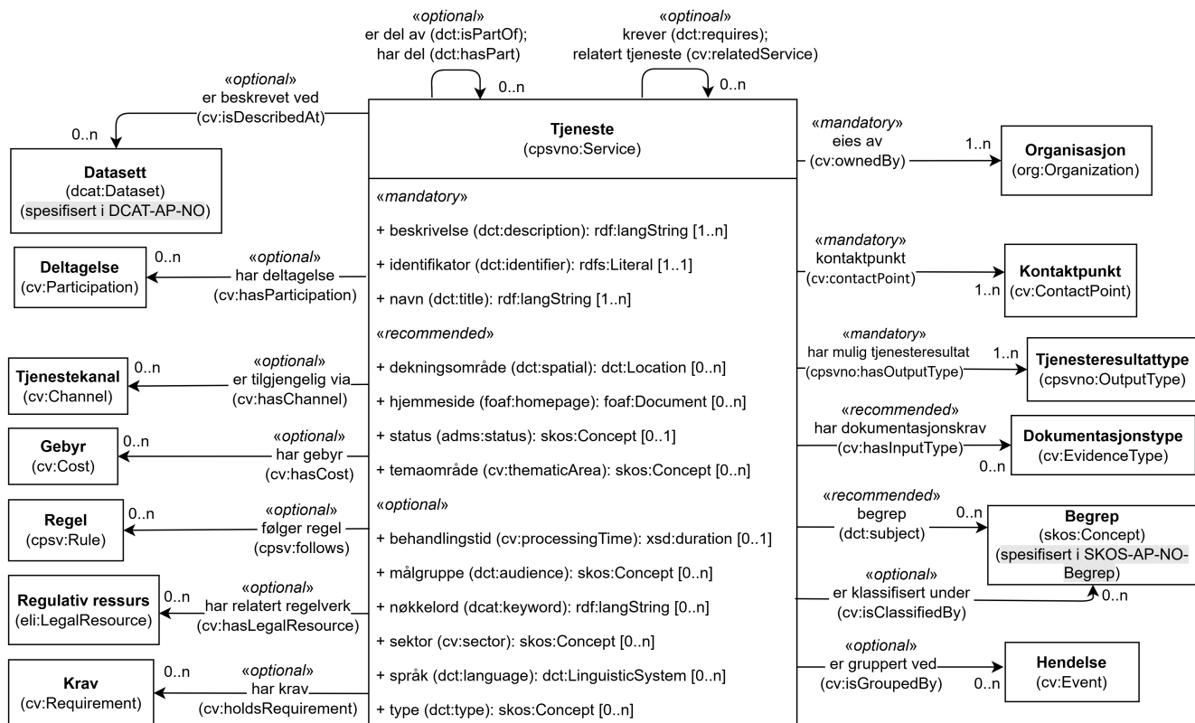
Figur 24. Klassen Tjeneste (cpsvno:Service) og klassene den refererer til.
