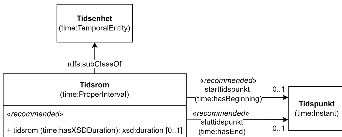
Figur 23. Klassen Tidsrom (time:ProperInterval) og klassene den refererer til.
