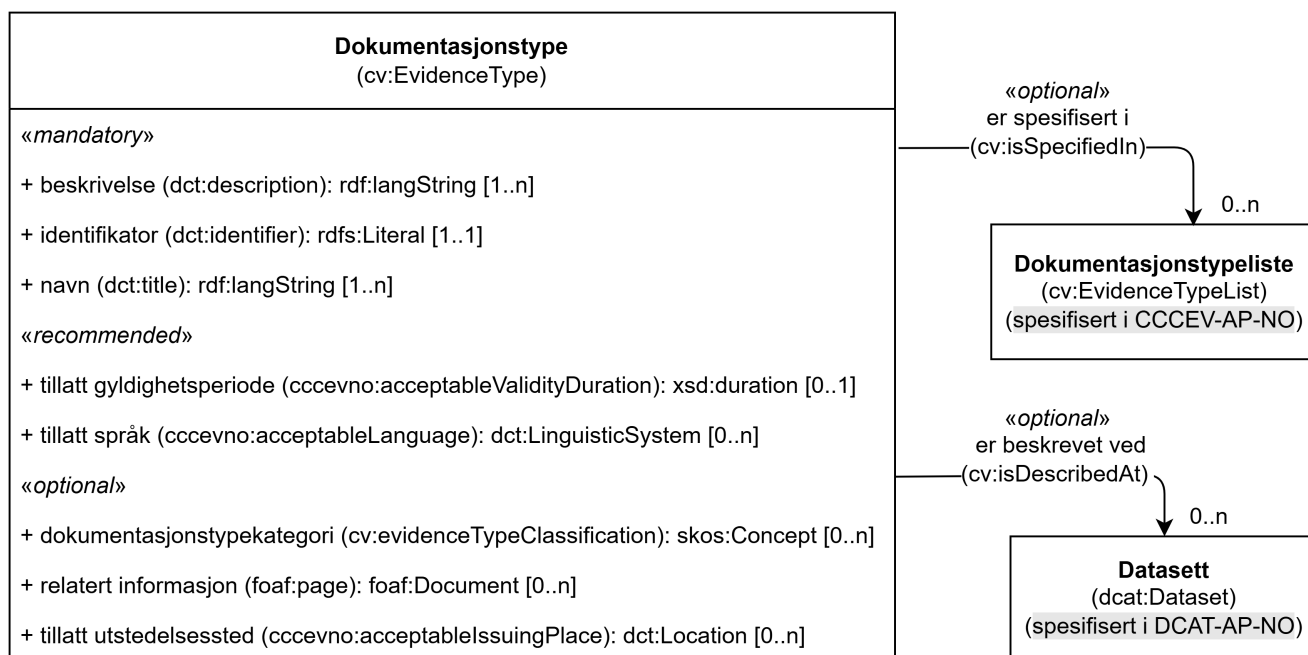
Figur 8. Klassen Dokumentasjonstype (cv:EvidenceType) og klassen den refererer til
