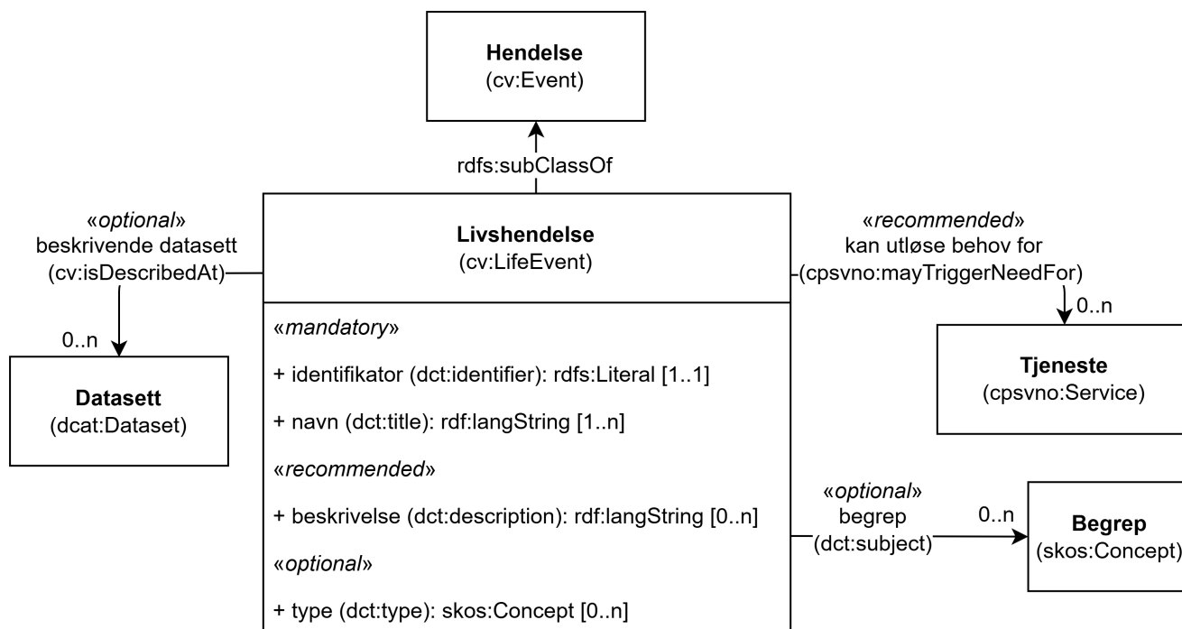
Figur 13. Klassen Livshendelse (cv:LifeEvent) og klassene den refererer til.
