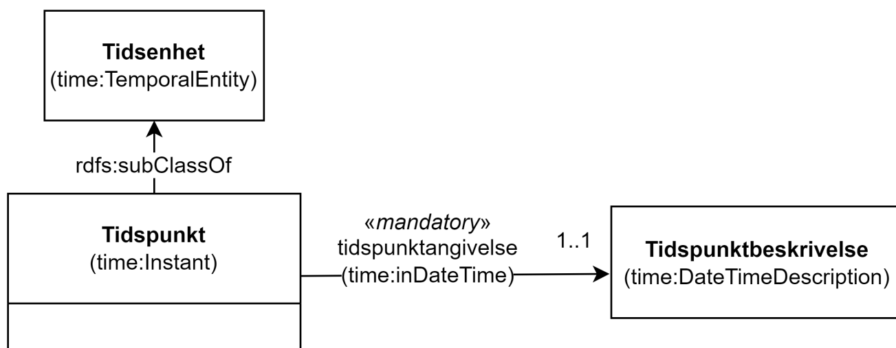
Figur 21. Klassen Tidspunkt (time:Instant) og klassene den refererer til.
