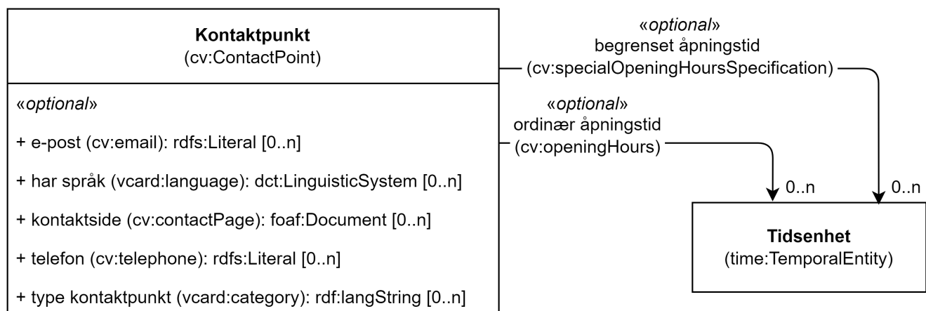
Figur 12. Klassen Kontaktpunkt (cv:ContactPoint) og klassen den refererer til.
