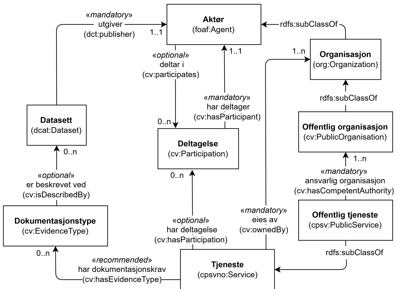
Figur 35. Tjeneste og Deltagelse.
