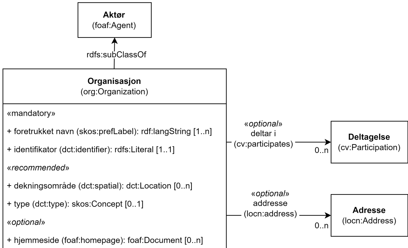
Figur 17. Klassen Organisasjon ( org:Organization ) og klassene den refererer til.
