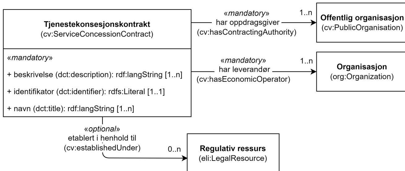
Figur 26. Klassen Tjenestekonsesjonskontrakt (cv:ServiceConcessionContract) og klassene den refererer til.
