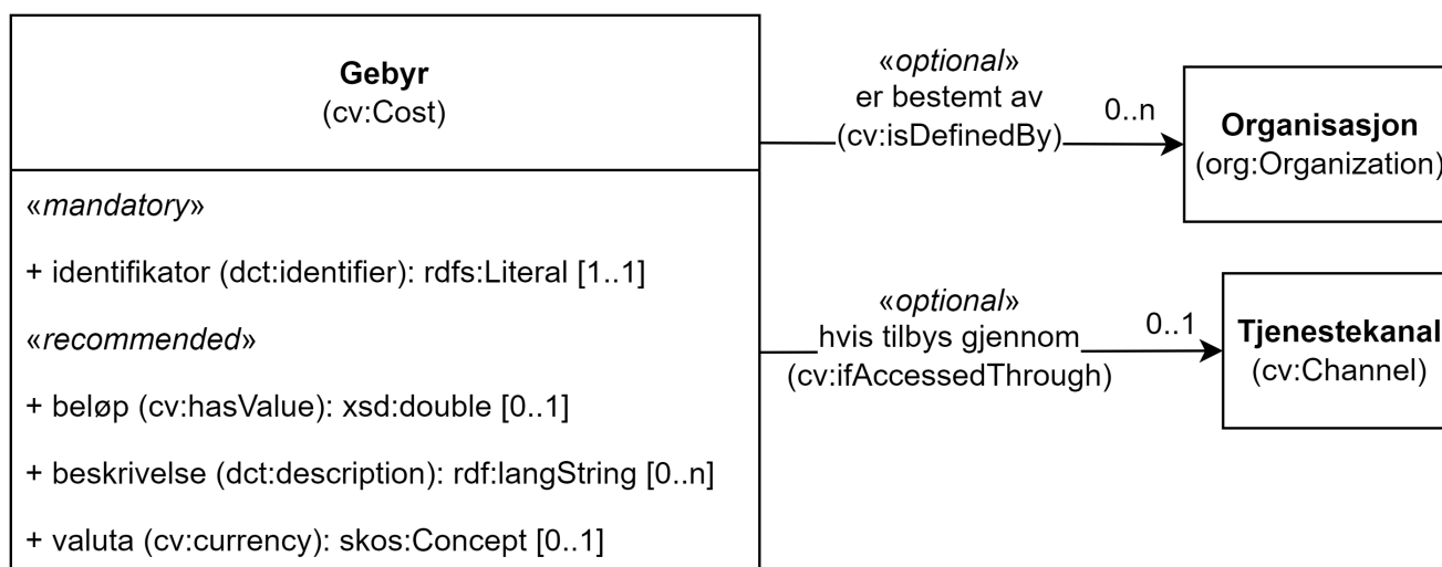
Figur 9. Klassen Gebyr (cv:Cost) og klassene den refererer til.
