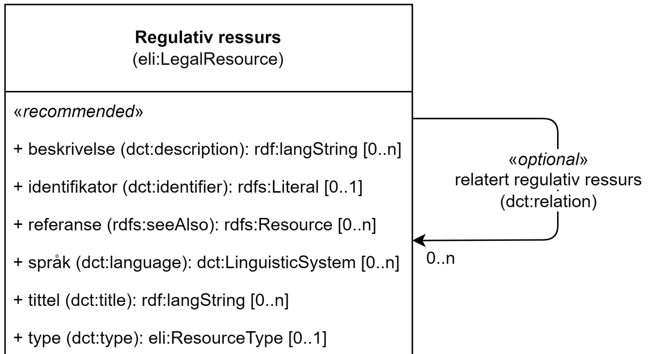
Figur 19. Klassen Regulativ ressurs (eli:LegalResource).
