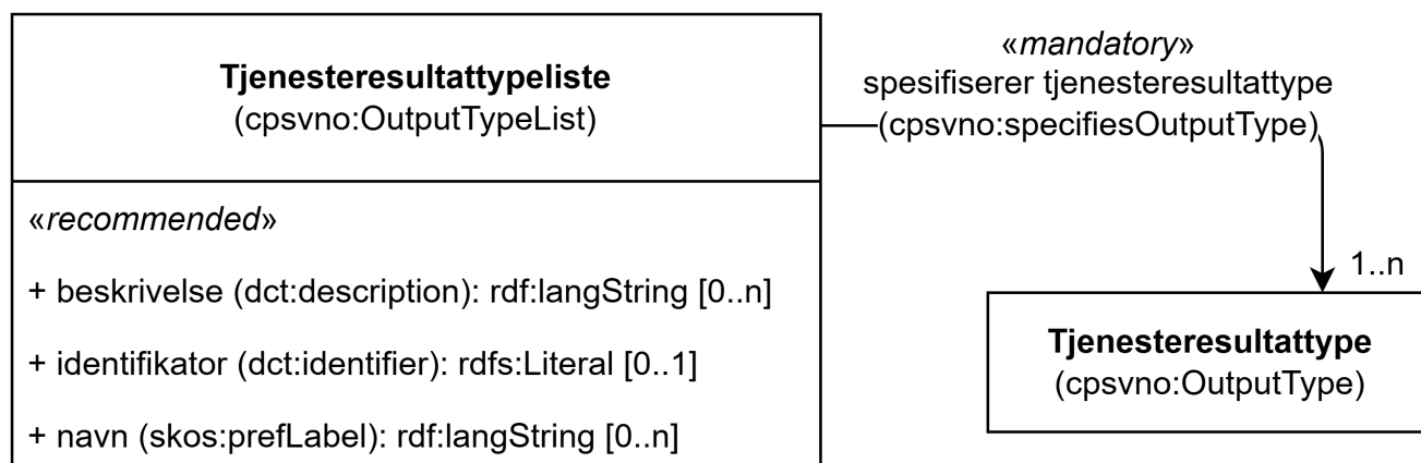
Figur 28. Klassen Tjenesteresultattypeliste (cpsvno:OutputTypeList) og klassen den refererer til
