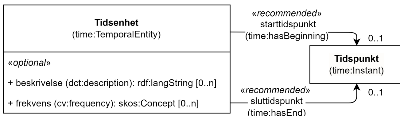
Figur 20. Klassen Tidsenhet (time:TemporalEntity) og klassen den refererer til.
