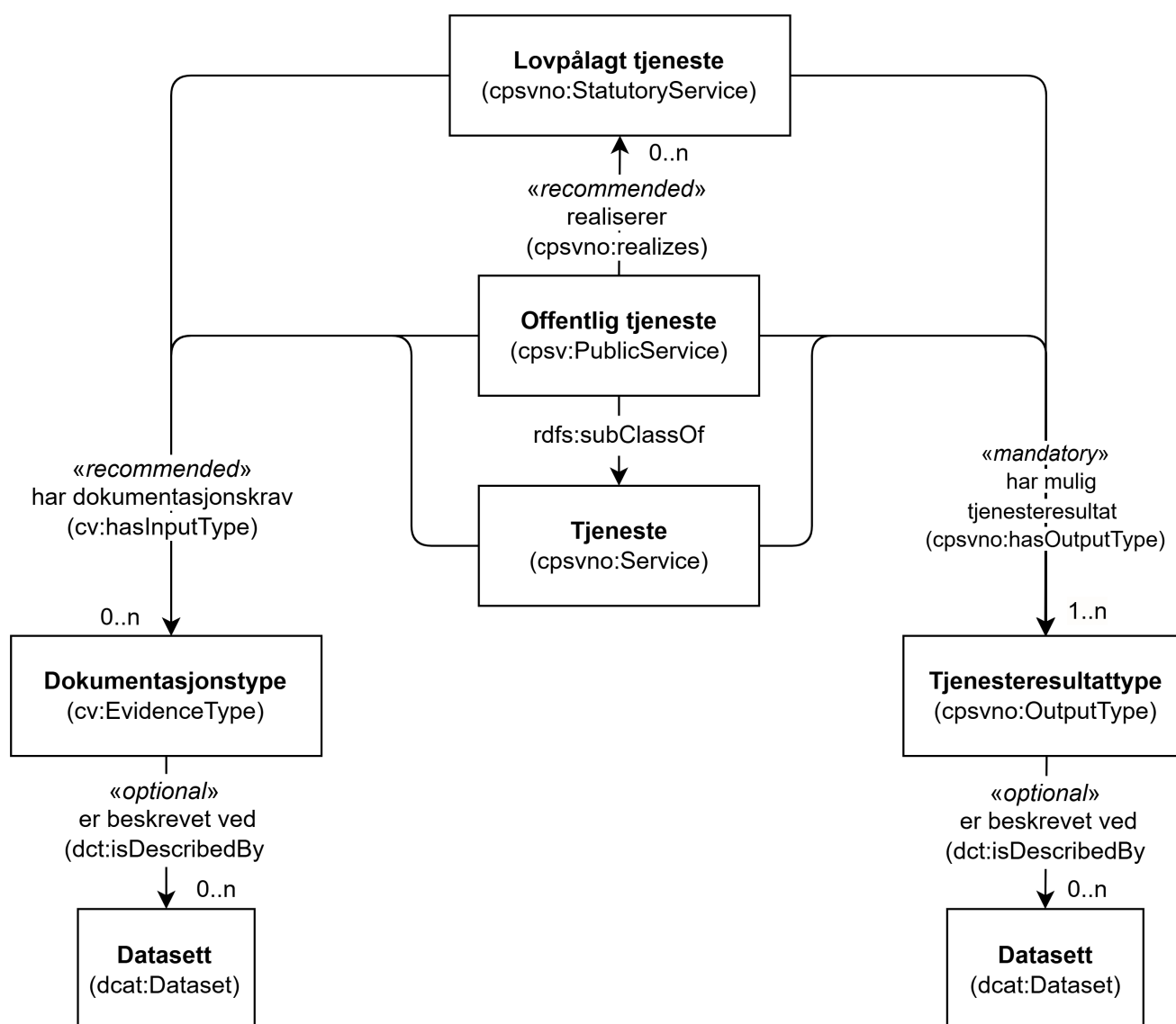
Figur 33. Tjeneste med påkrevd dokumentasjon og mulig tjenesteresultat som er del av datasett.
