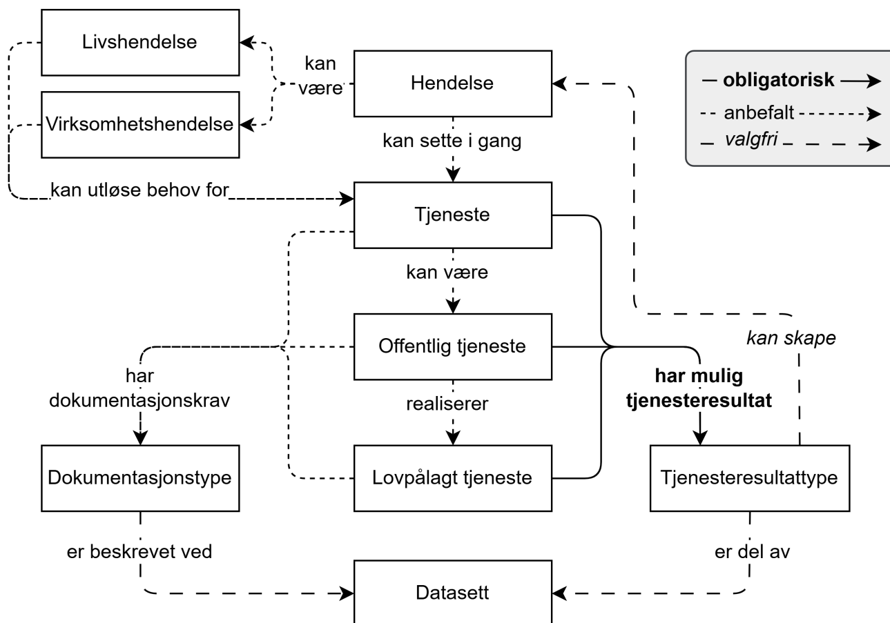
Figur 2. Forenklet fremstilling av CPSV-AP-NO.
