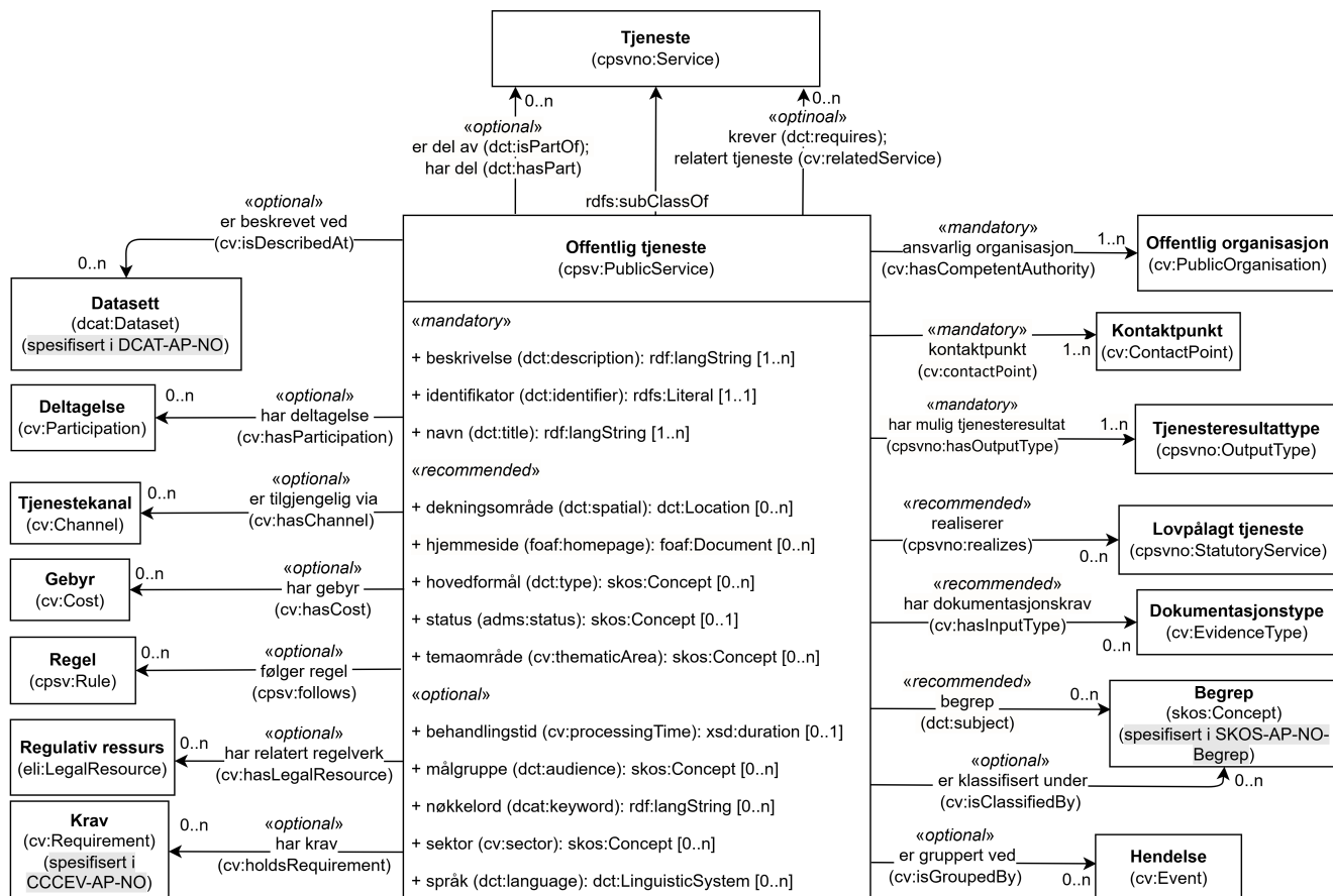
Figur 16. Klassen Offentlig tjeneste (cpsv:PublicService) og klassene den refererer til.
