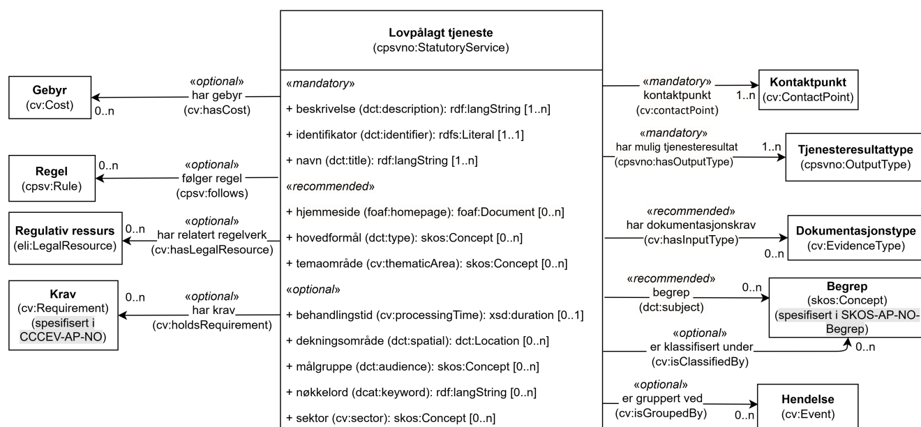
Figur 14. Klassen Lovpålagt tjeneste (cpsvno:StatutoryService) og klassene den refererer til.
