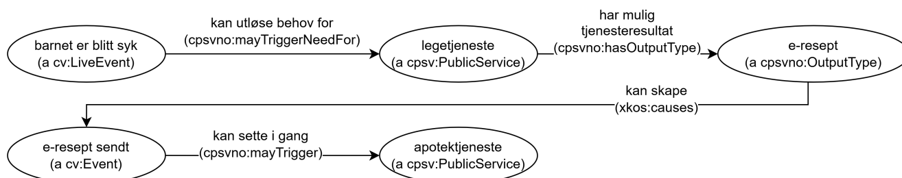
Figur 31. Eksempel på bruk av CPSV-AP-NO til å beskrive deler av livshendelsen "Alvorlig sykt barn".
