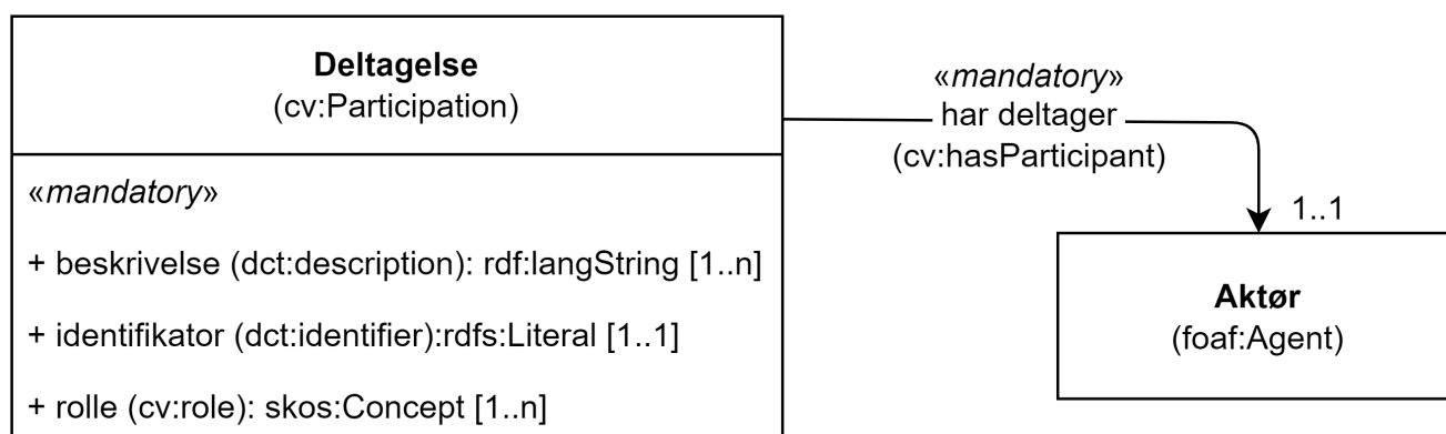
Figur 7. Klassen Deltagelse (cv:Participation) og klassen den refererer til.
