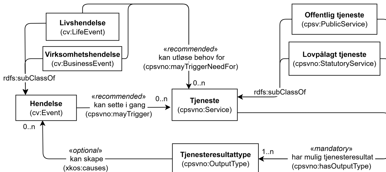
Figur 30. Klasser og egenskaper for beskrivelse av en tjenestekjede.
