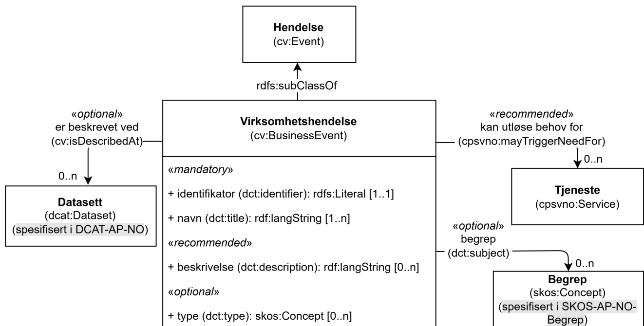
Figur 29. Klassen Virksomhetshendelse (cv:BusinessEvent) og klassene den refererer til.
