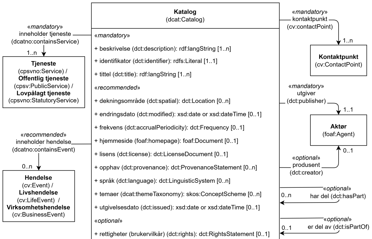
Figur 11. Klassen Katalog (dcat:Catalog) og klassene den refererer til.
