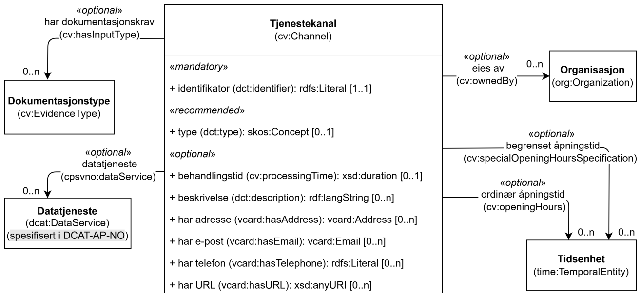
Figur 25. Klassen Tjenestekanal (cv:Channel) og klassene den refererer til.
