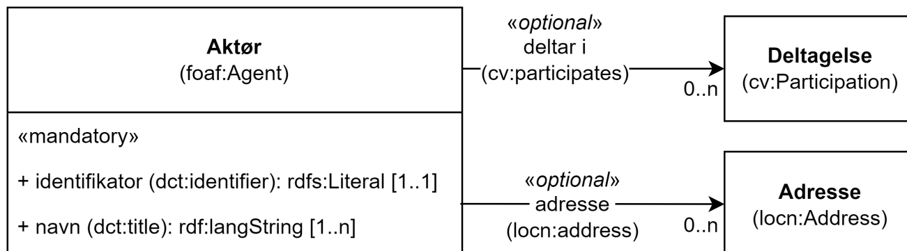
Figur 6. Klassen Aktør (foaf:Agent) og klassene den refererer til.
