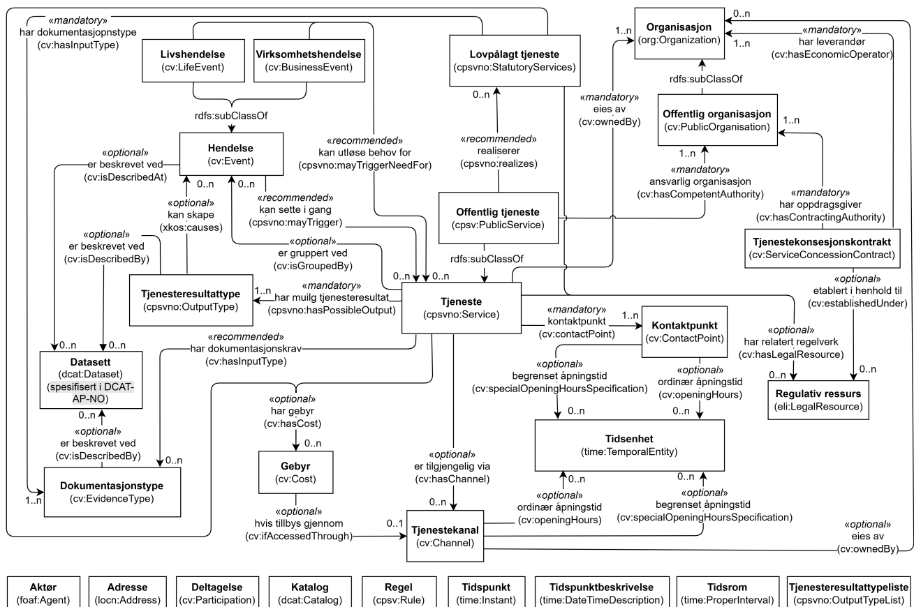
Figur 4. Klassene i CPSV-AP-NO.
