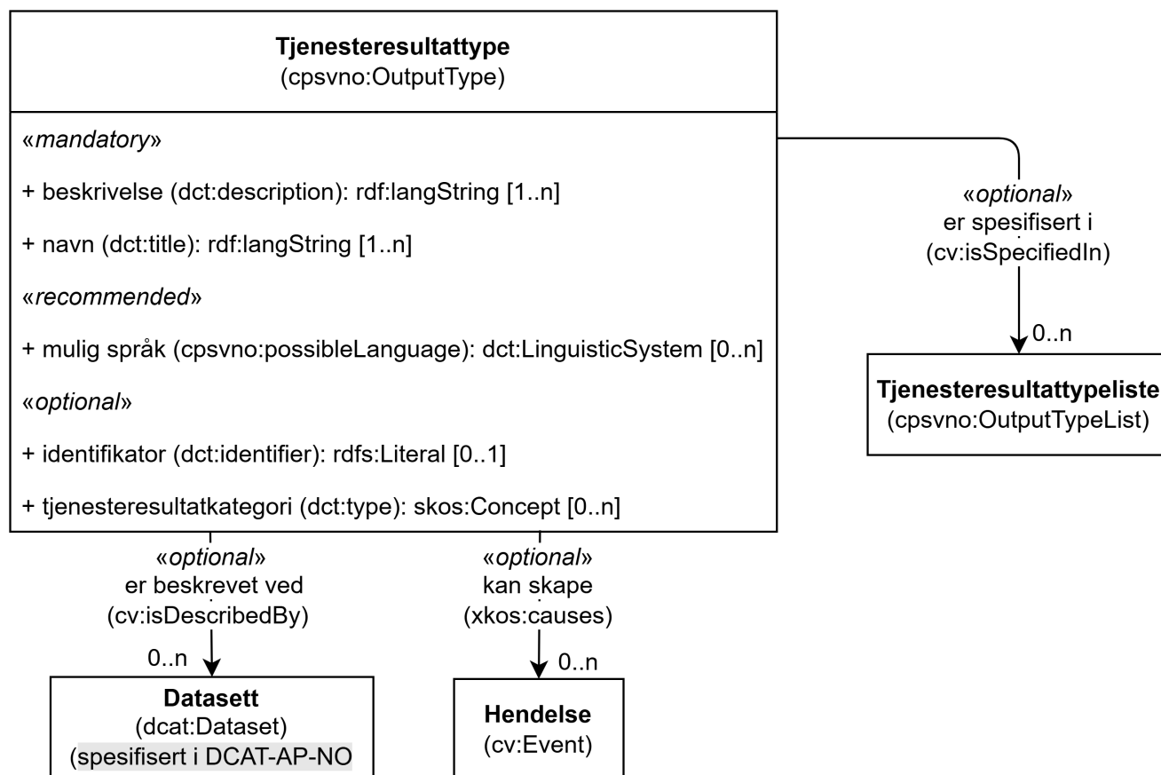
Figur 27. Klassen Tjenesteresultattype (cpsvno:OutputType) og klassene den refererer til.
