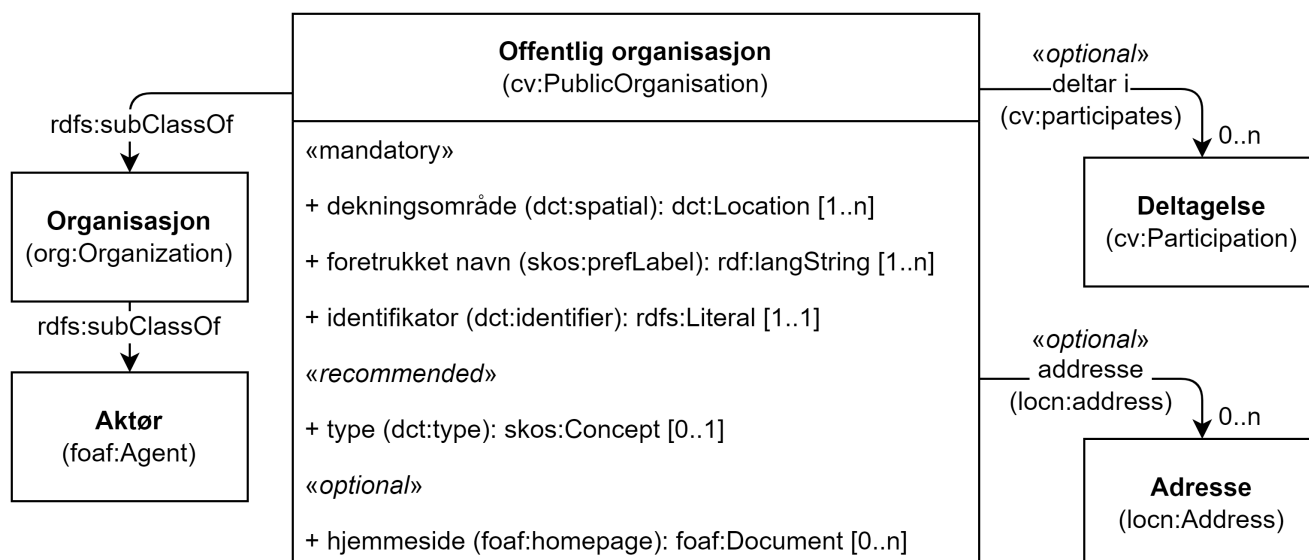
Figur 15. Klassen Offentlig organisasjon (cv:PublicOrganisation) og klassene den refererer til.
