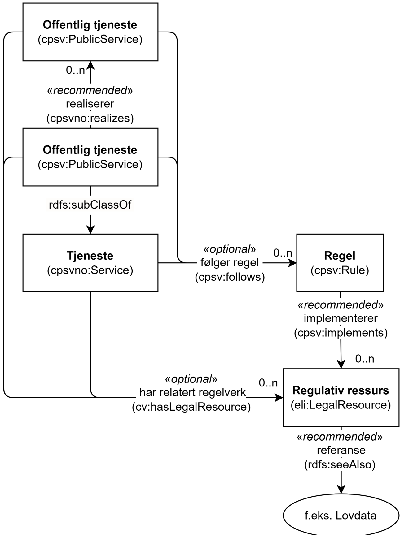
Figur 34. Tjeneste og regelverk.
