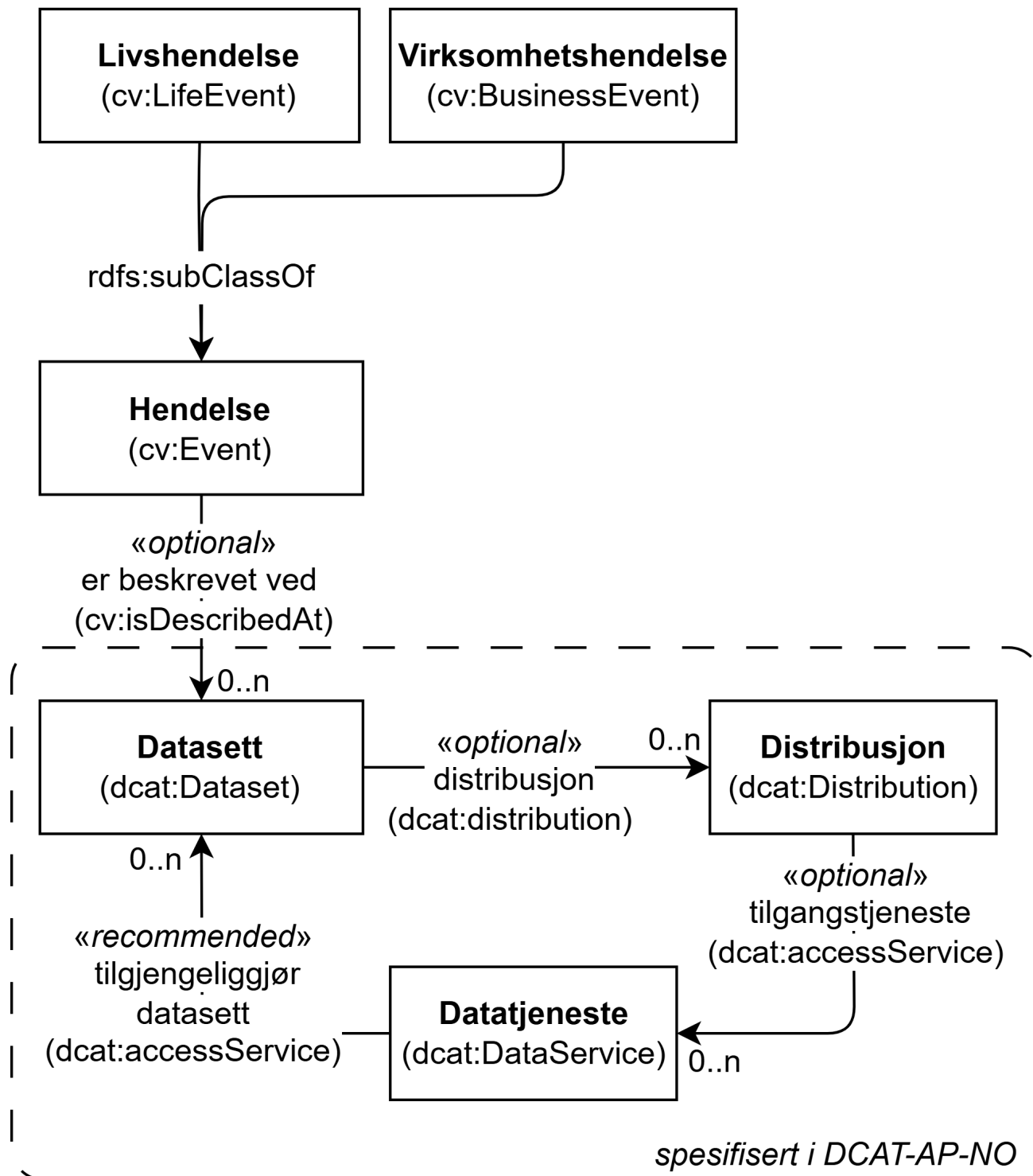
Figur 32. Hendelse og Distribusjon.
