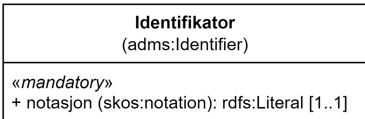
Figur 9. Klassen Identifikator.
