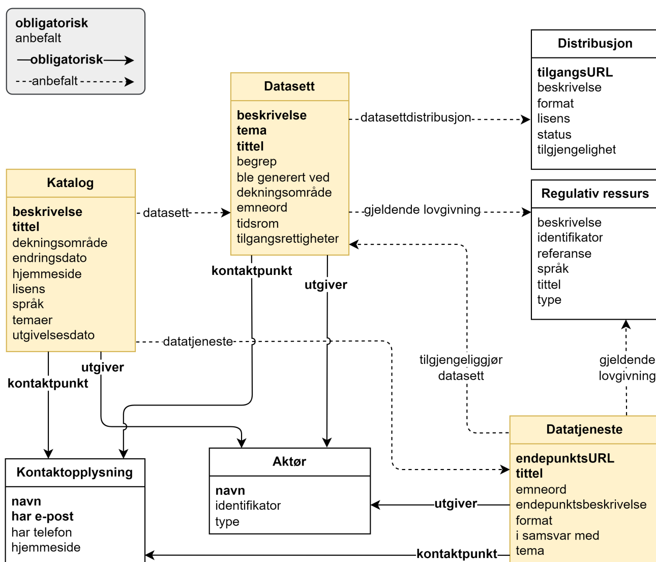
Figur 1. Forenklet fremstilling av noen av kravene i DCAT-AP-NO.
