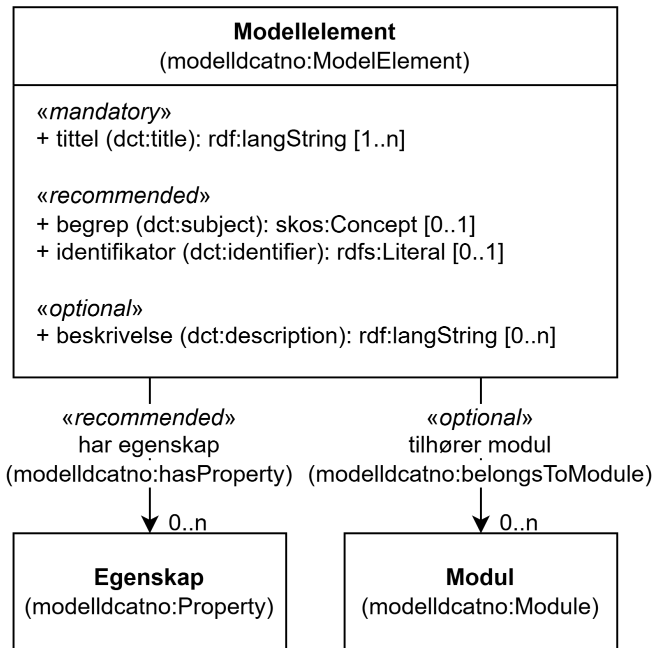
Figur 23. Klassen Modelelement ( modelldcatno:ModelElement ) og klassene den refererer til
