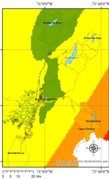
b) Sismo 475 años
