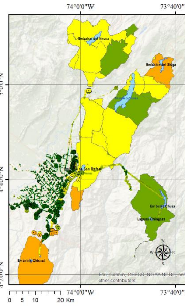
h) Incendios forestales
