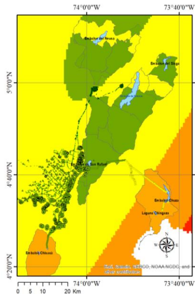
a) Sismo 225 años
