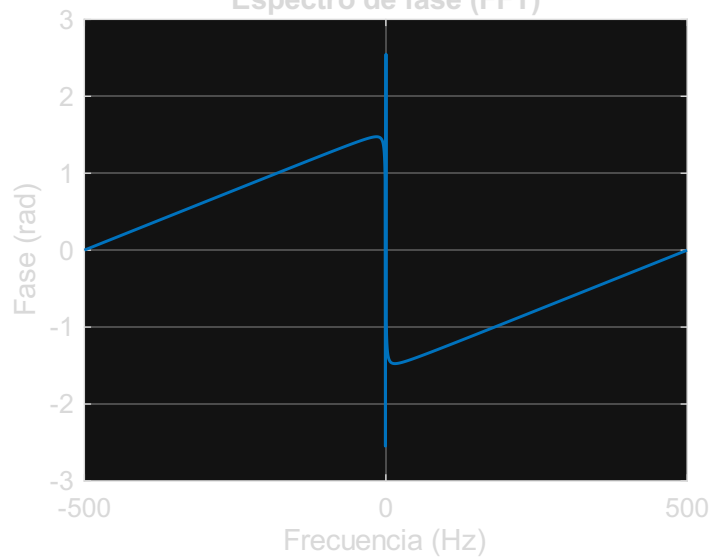
Espectro de fase (FFT)
