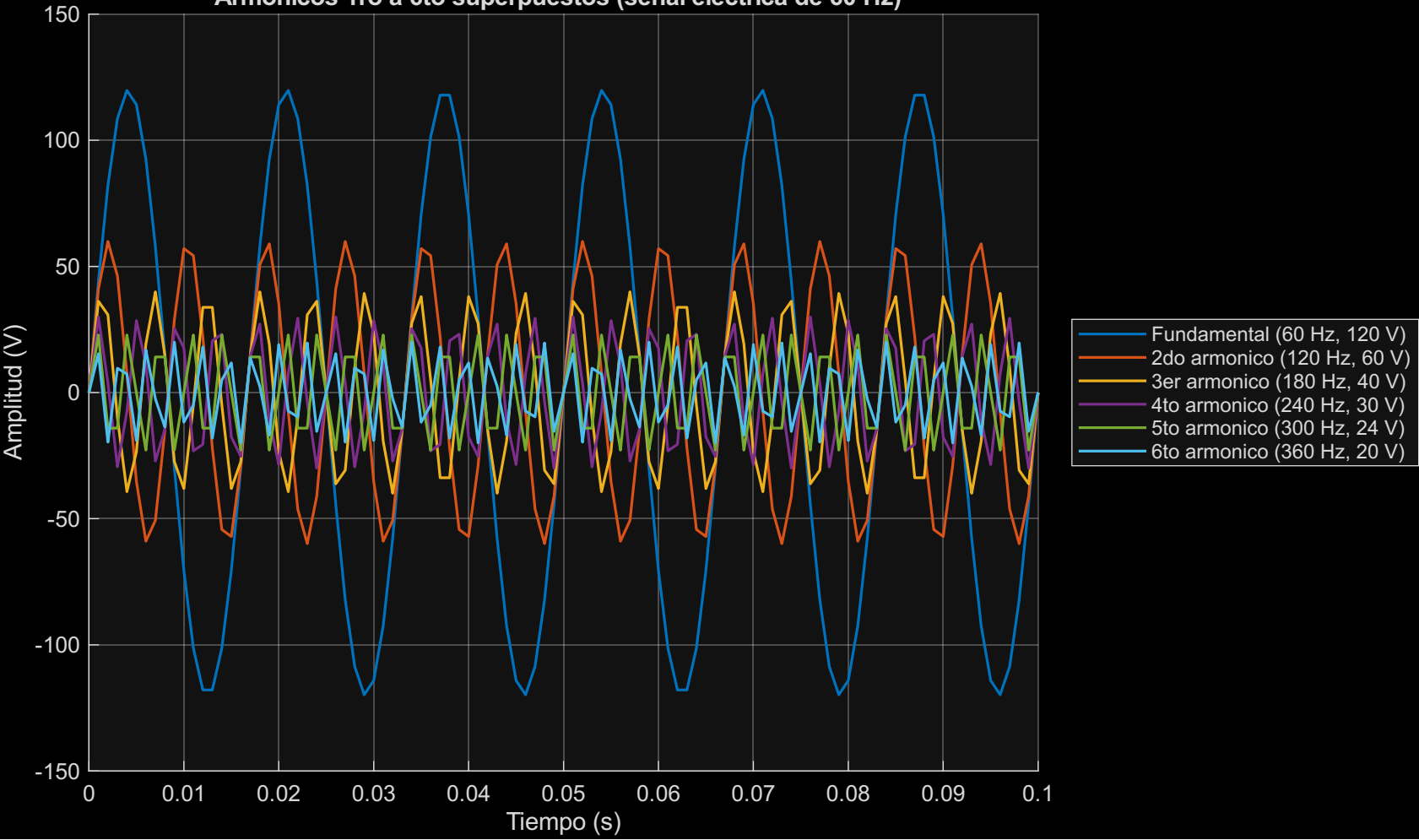
Armonicos 1ro a 6to superpuestos (senal electrica de 60 Hz)
