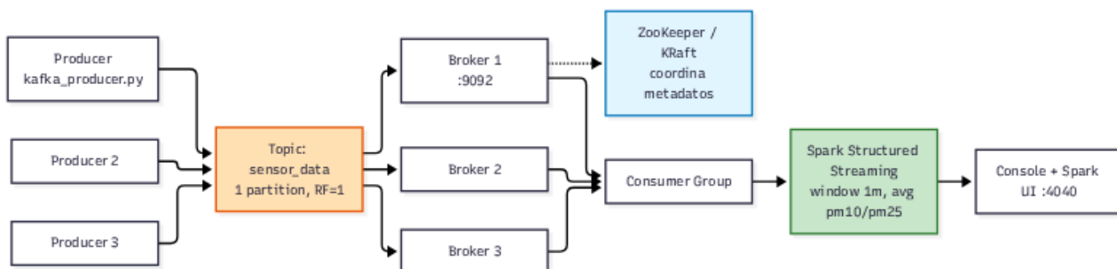
Captura Mermaid 1: Arquitectura Kafka + Spark
