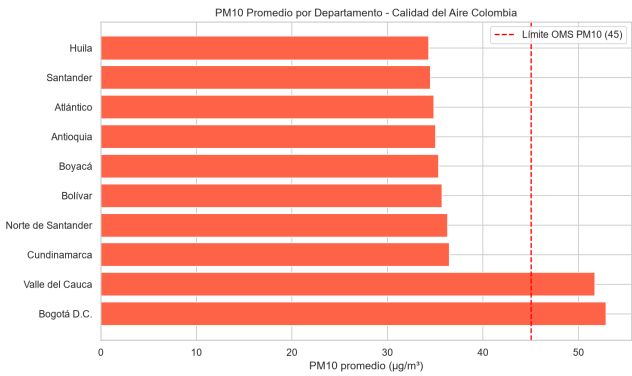
Fig. 1: Ranking PM10 por departamento
