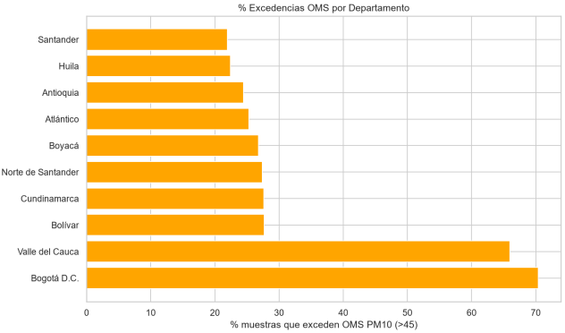
Fig. 4: % Excedencia OMS por depto
