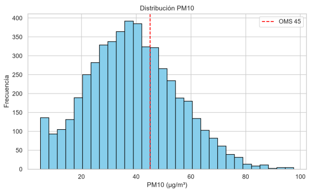
Fig. 2: Histograma PM10 (OMS 45)
