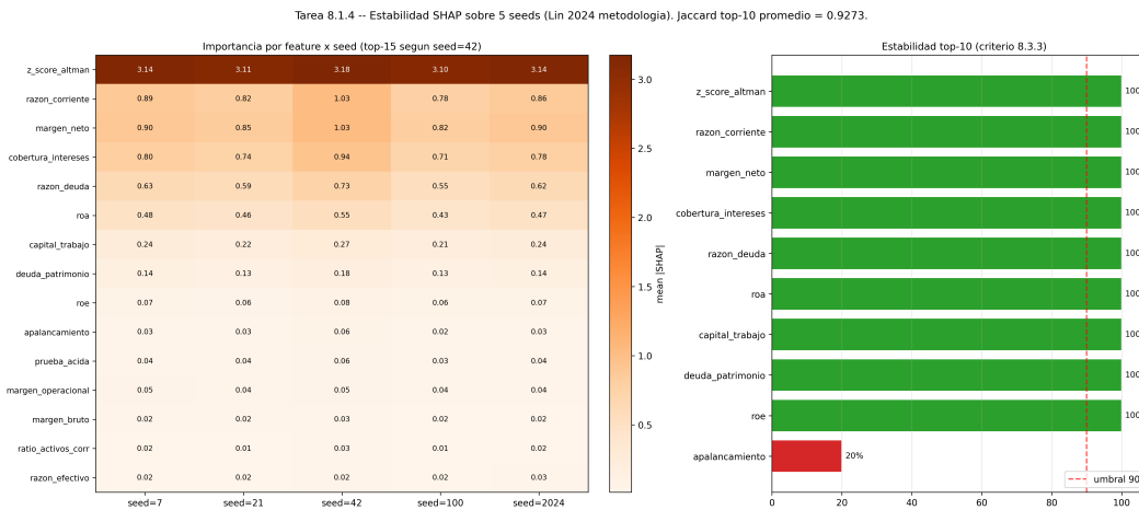
Figura 15: Estabilidad del top-10 SHAP sobre cinco semillas aleatorias {7, 21, 42, 100, 2024}. Top-3 estable al 100%; Jaccard promedio = 0,927.
