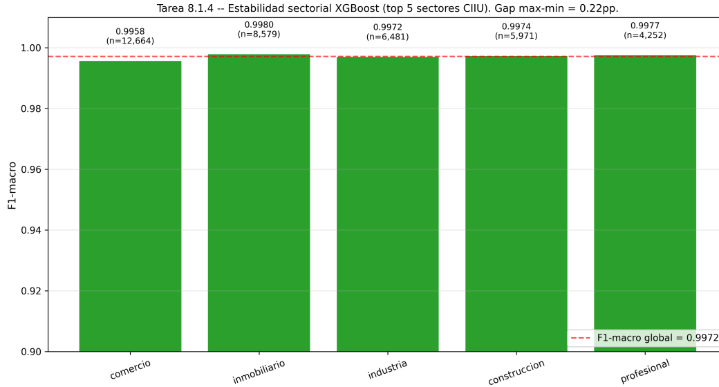
Figura 14: Estabilidad de F1-macro por sector CIU sobre el conjunto de test (top 5 sectores). Gap máximo-mínimo = 0,22 pp.
