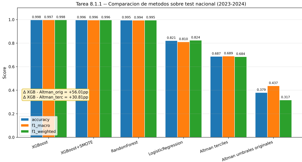
Figura 13: Comparación de F1-macro entre XGBoost y los métodos clásicos sobre el conjunto de test nacional ( n = 50\,957 ). XGBoost supera a Altman puro por +56,0 pp.
