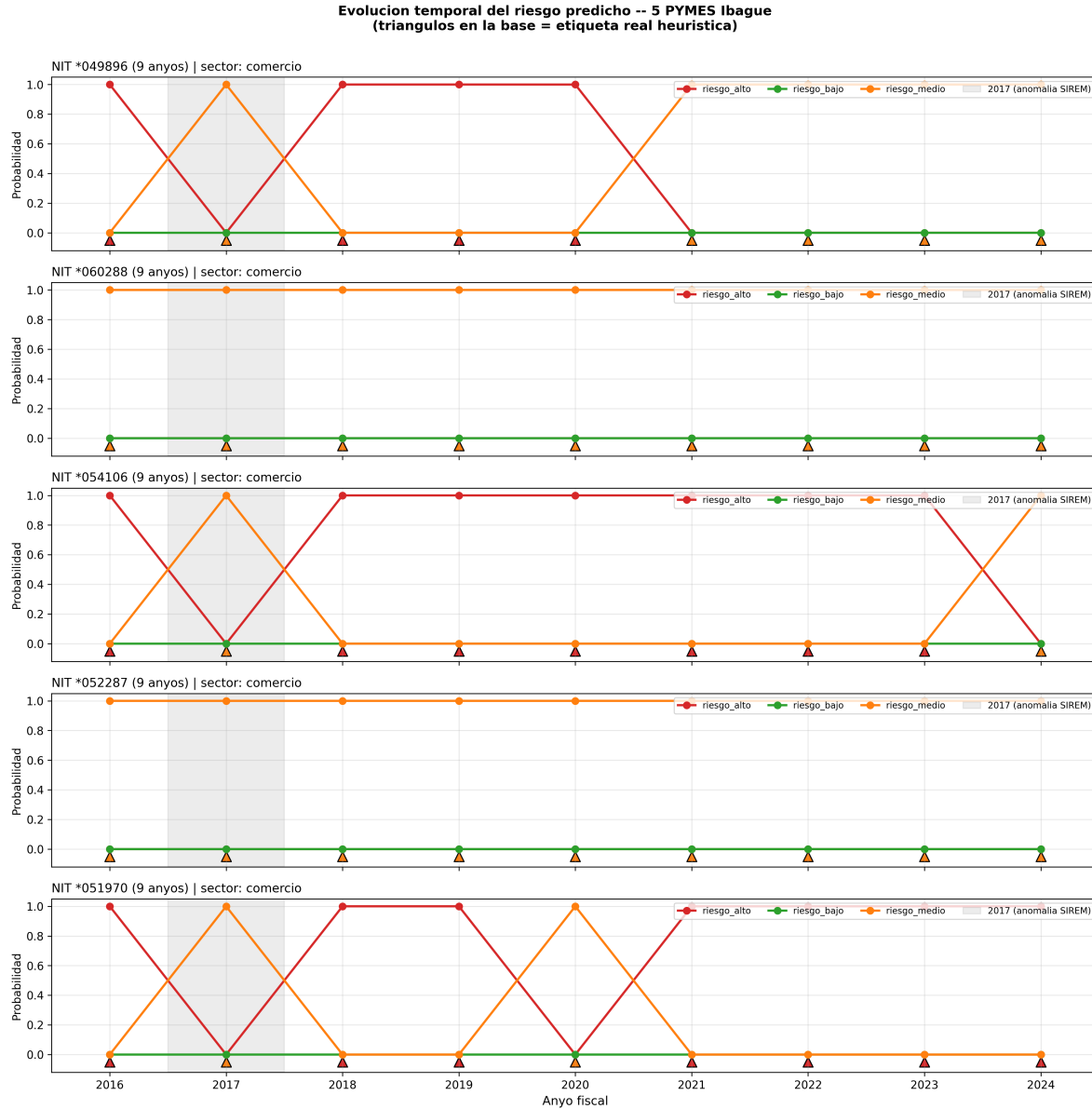
Figura 12: Evolución temporal de la clasificación de riesgo (real vs. predicho) para cinco PYMES de Ibagué con cobertura completa de 9 años.
