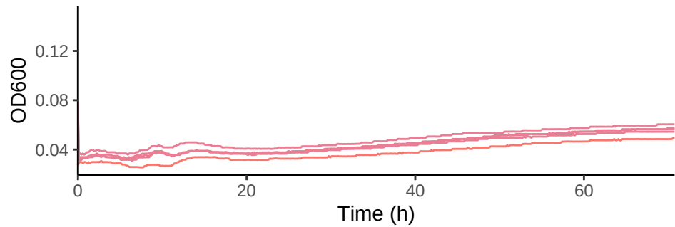
DSS3 in DMSP 4 mM C with Kan 50
