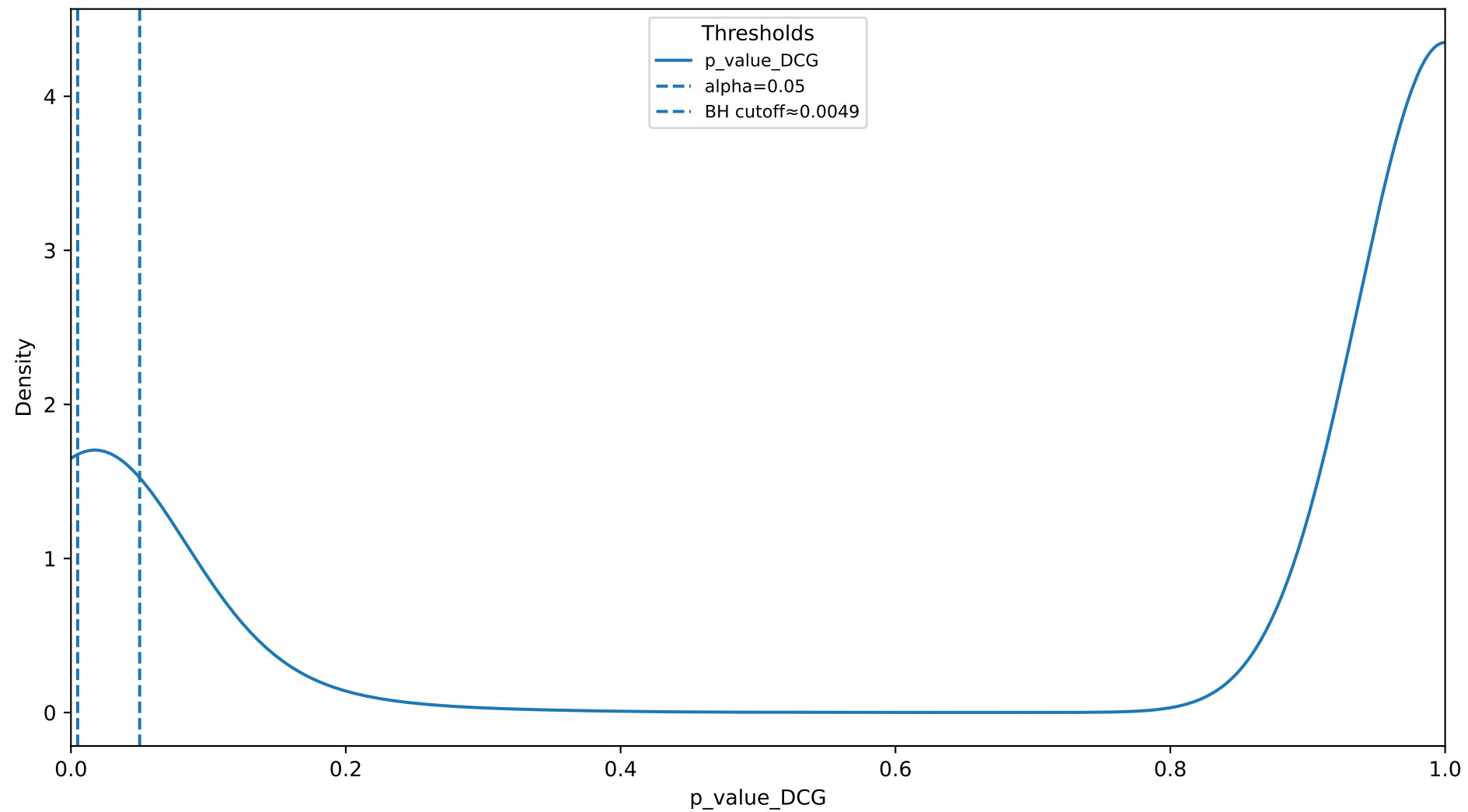
KDE of DCG p-values (string_min700)
