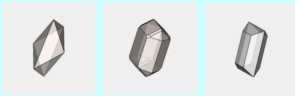
typische Kristallformen
