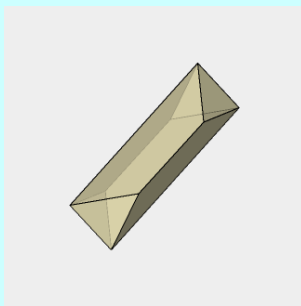
Kristallformen (Bsp.)
