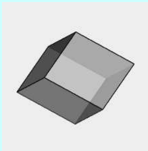
typische Kristallformen
