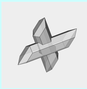
typische Kristallformen und Zwillinge
